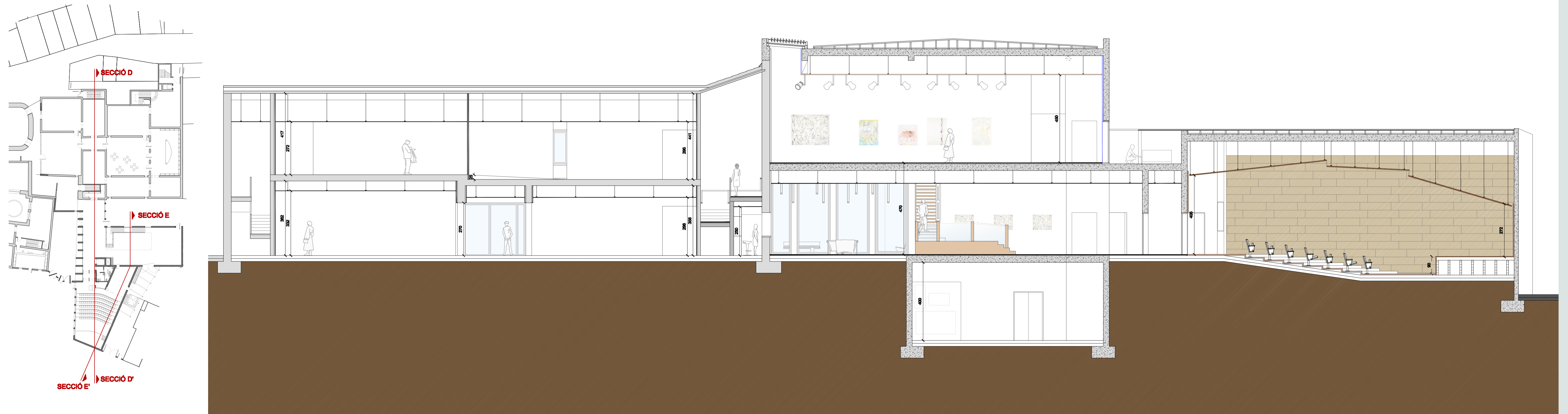
SECCIÓ D-D'
