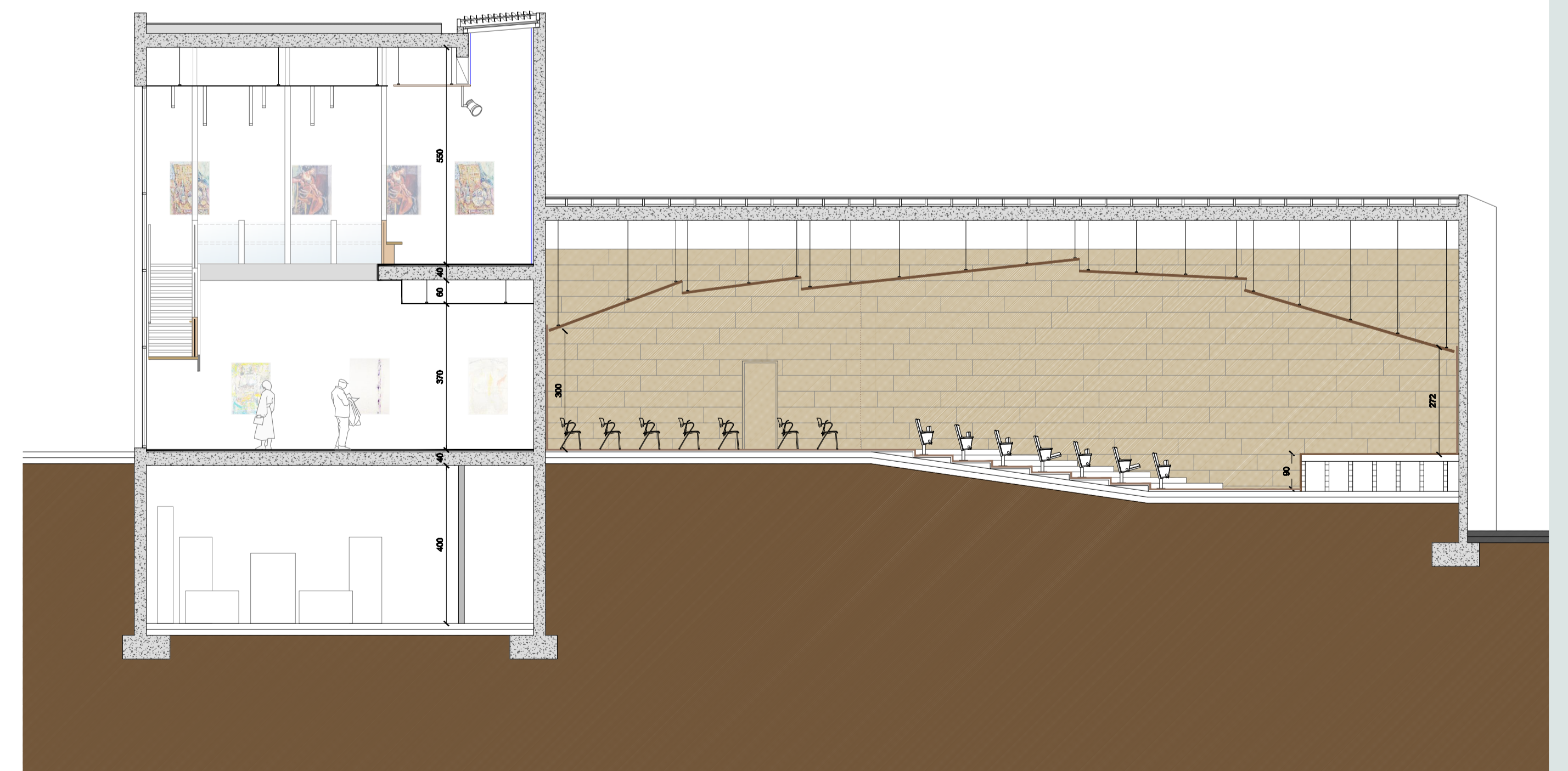
SECCIÓ E-E'
