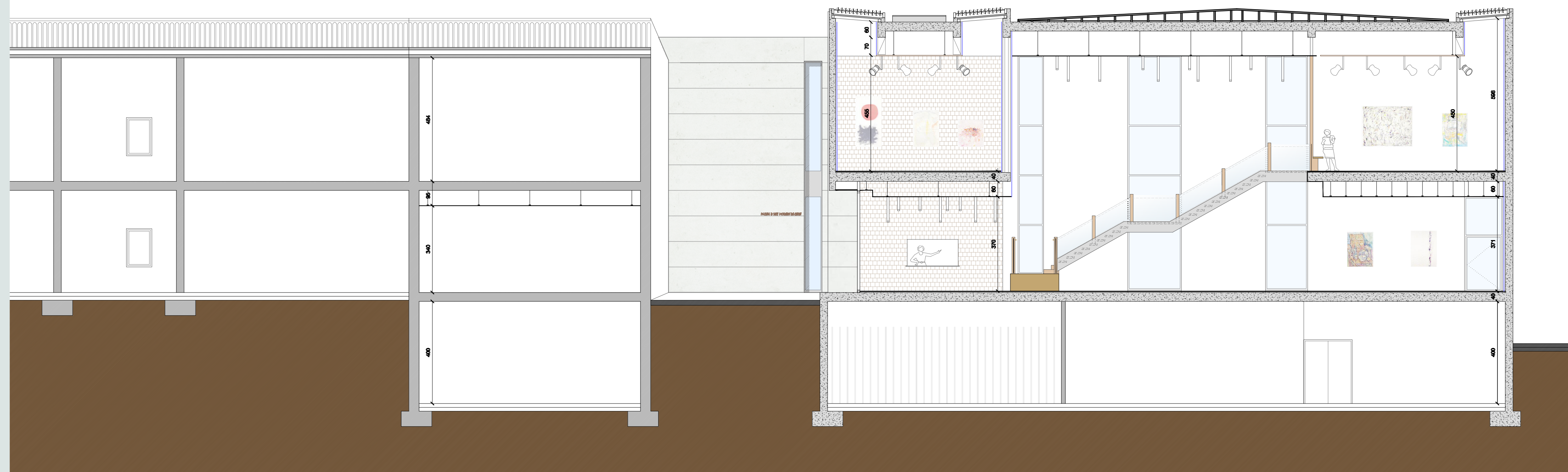
SECCIÓ C-C'
