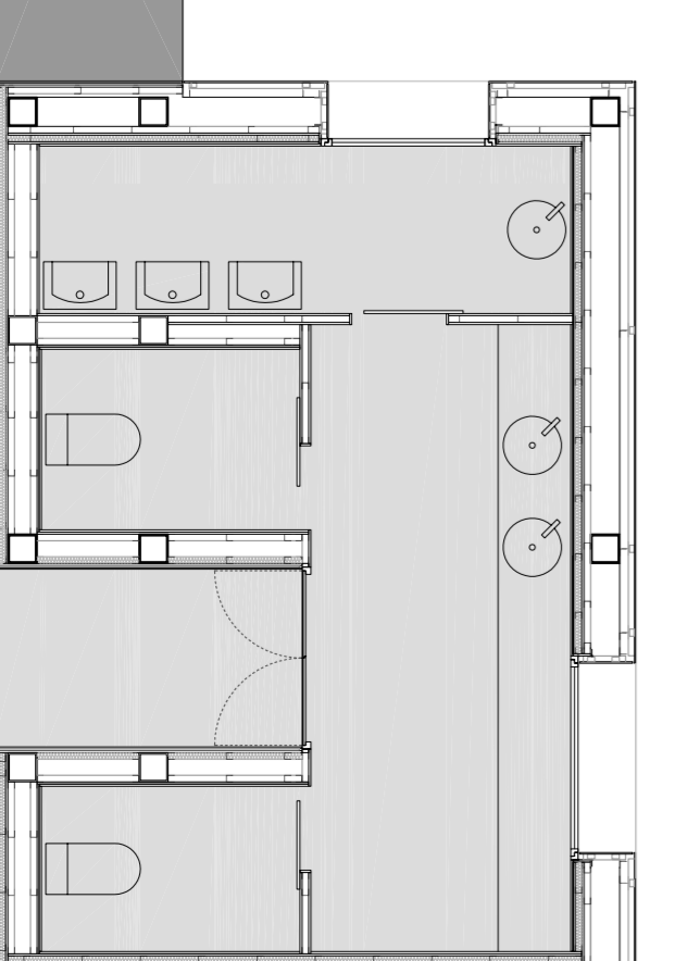
LAVABO (e/v/50)
