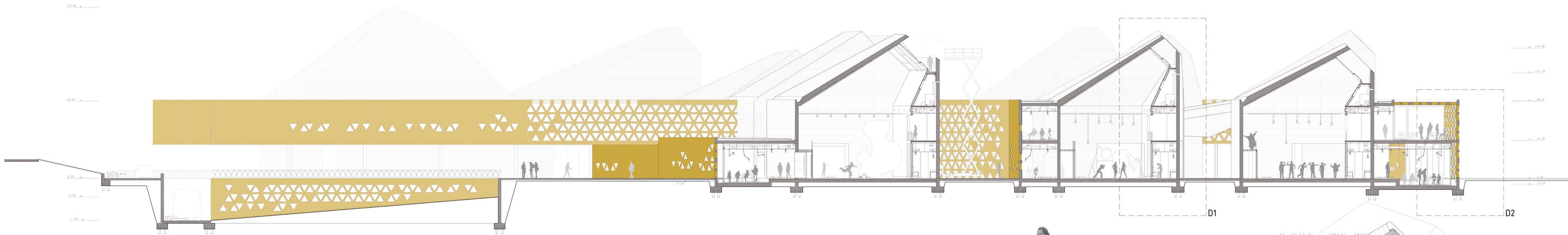
01. SECCION LONGITUDINAL A-A' 1/100 Espacios de trabajo; talleres y laboratorios. Sistema de iluminación cenital y mantenimiento.
