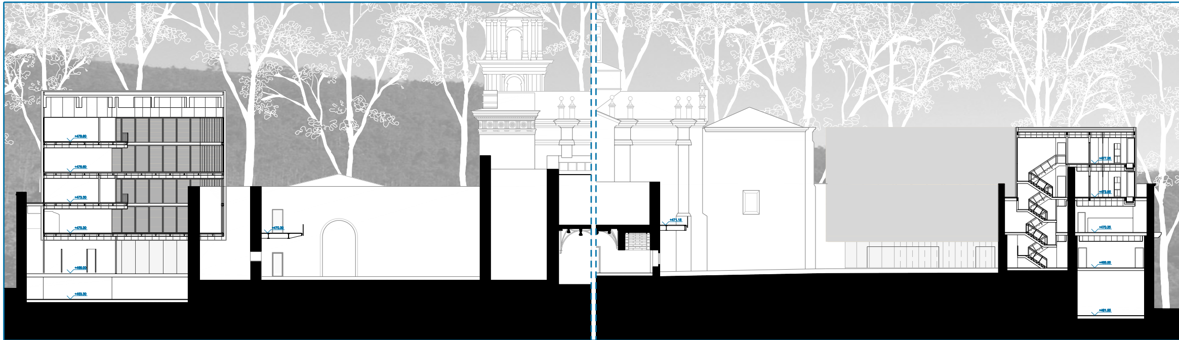
SECCIÓ 12-12', E:1/200
