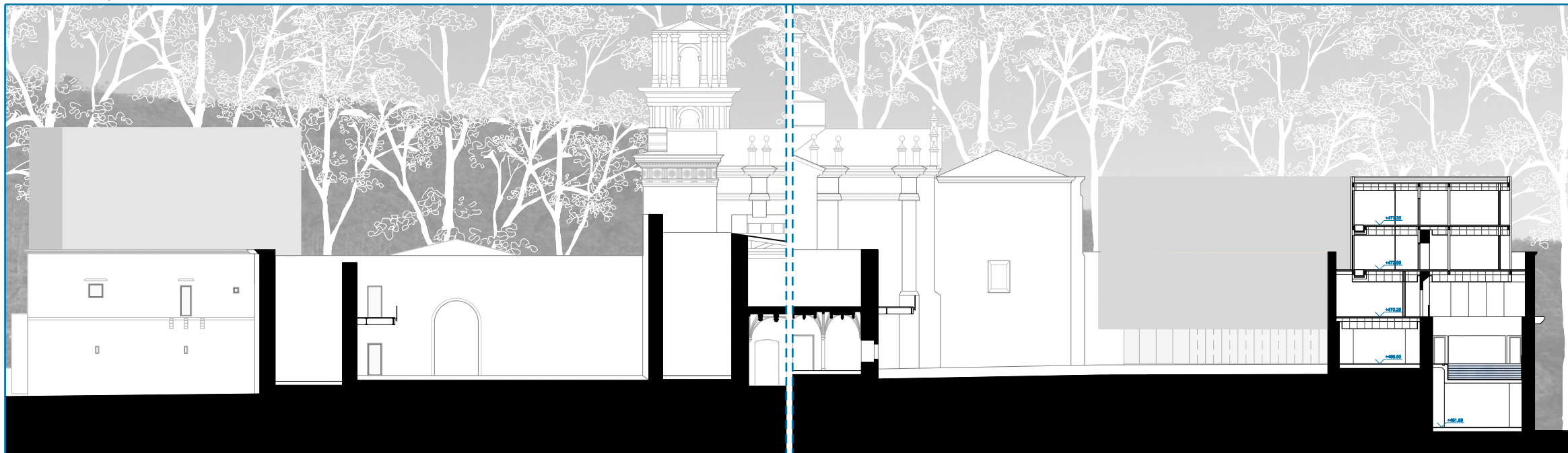
SECCIÓ 13-13', E:1/200
