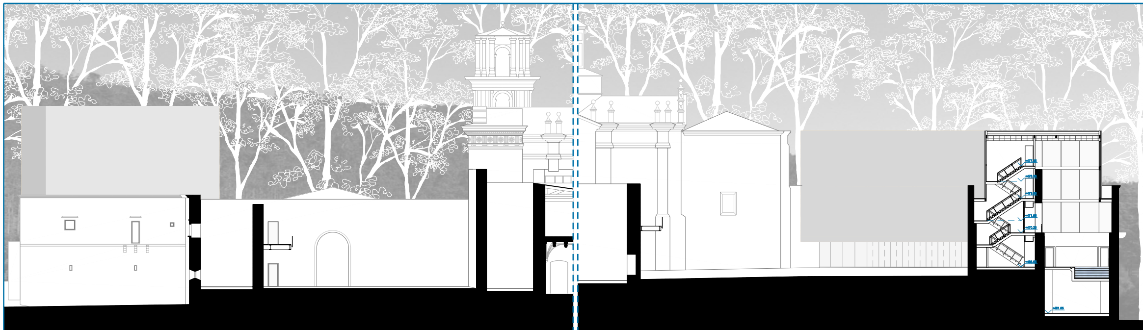
SECCIÓ 14-14', E:1/200
