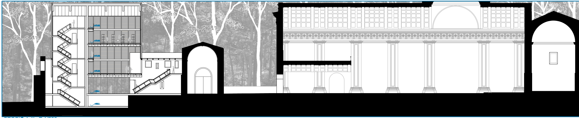
SECCIÓ 1-1', E:1/200
