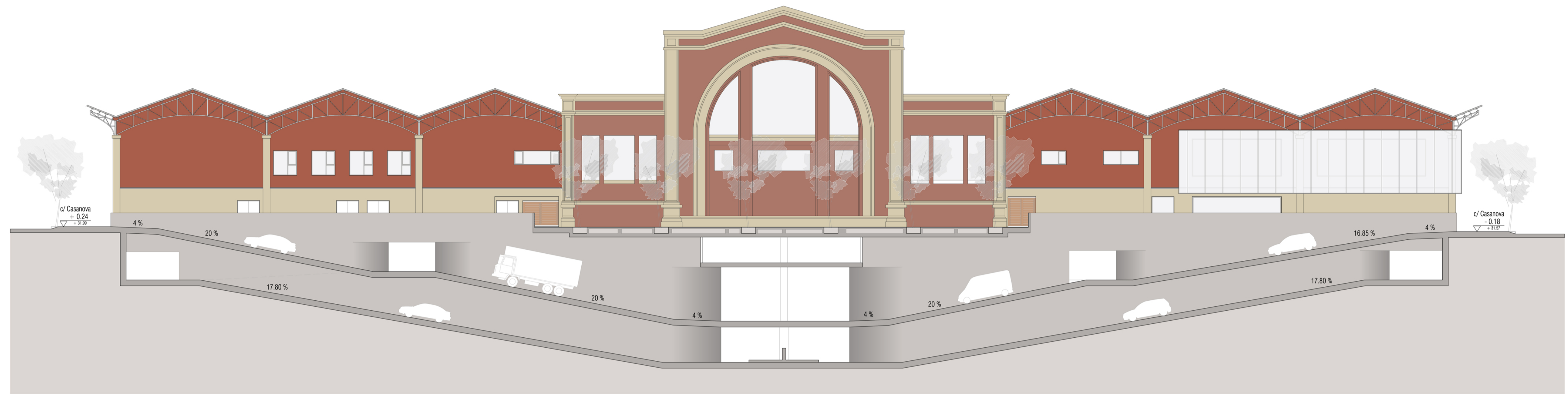
Secció A-A'
