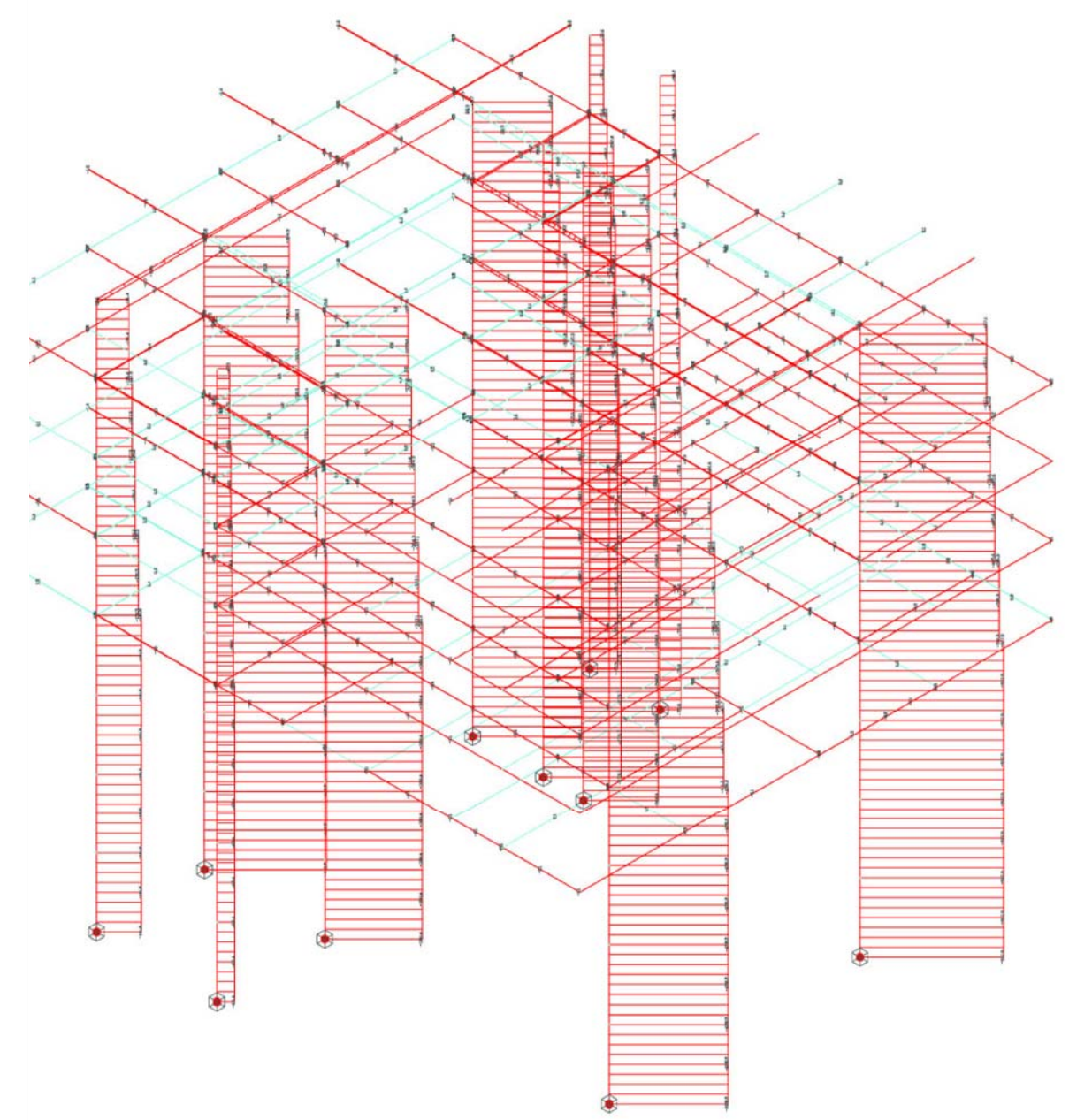
Diagrama d' AXILS dels pilars i pantalles de formigó: Diagrama d'axil a compressió.
