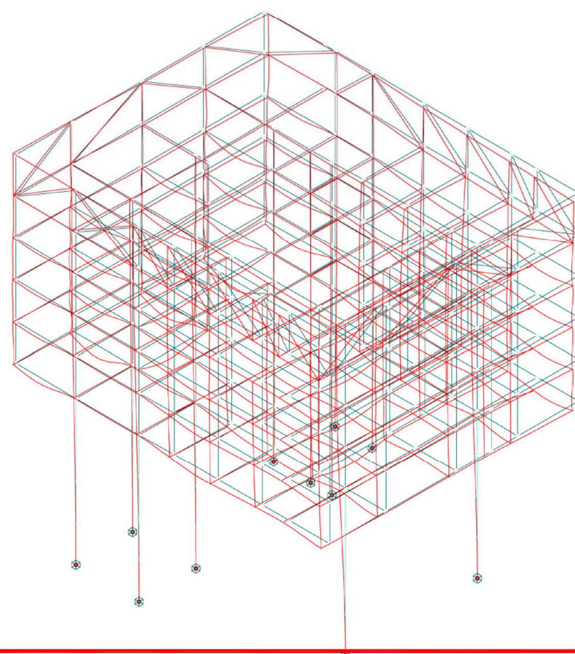
DEFORMACIÓ d'un dels subgrups. S'ha dimensionat l'estructura de manera que la fletxa no superés 1cm ja que això provocaria grans esforços sobre els envans.
