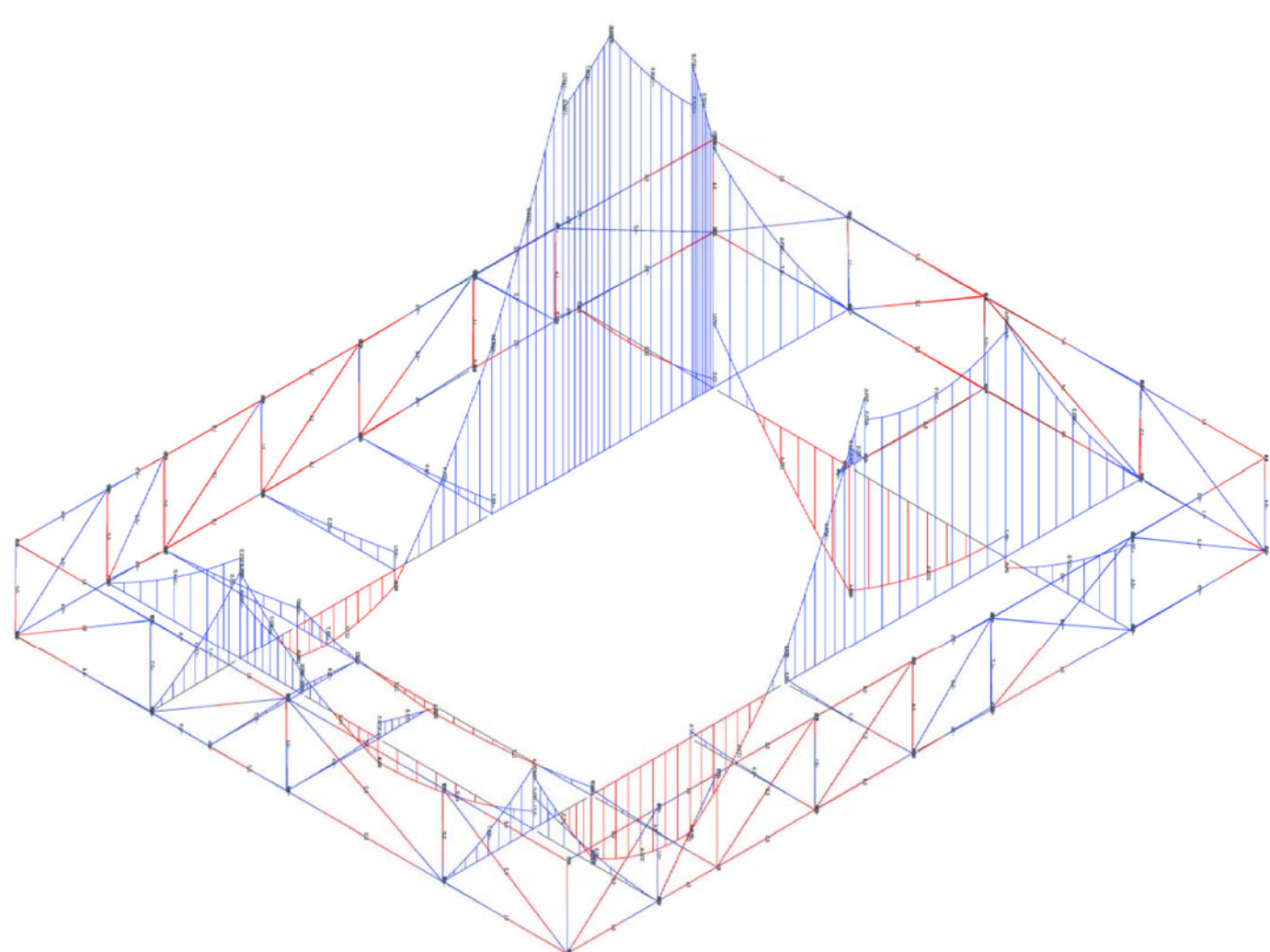
Diagrama de MOMENTS de la planta plataforma
