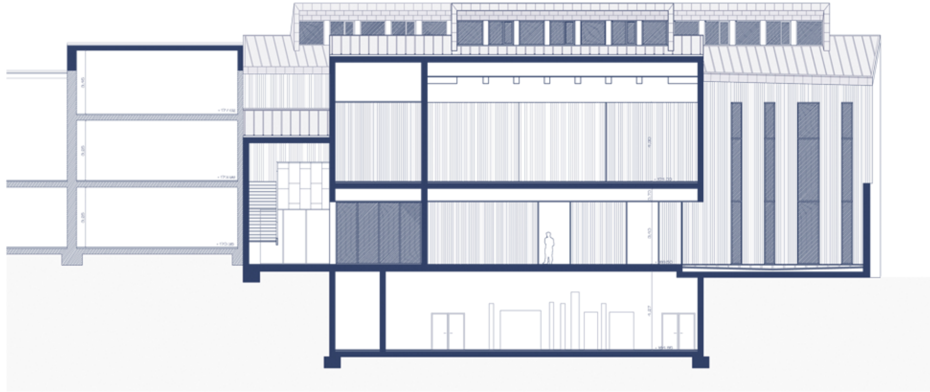
SECCIÓN G G'
