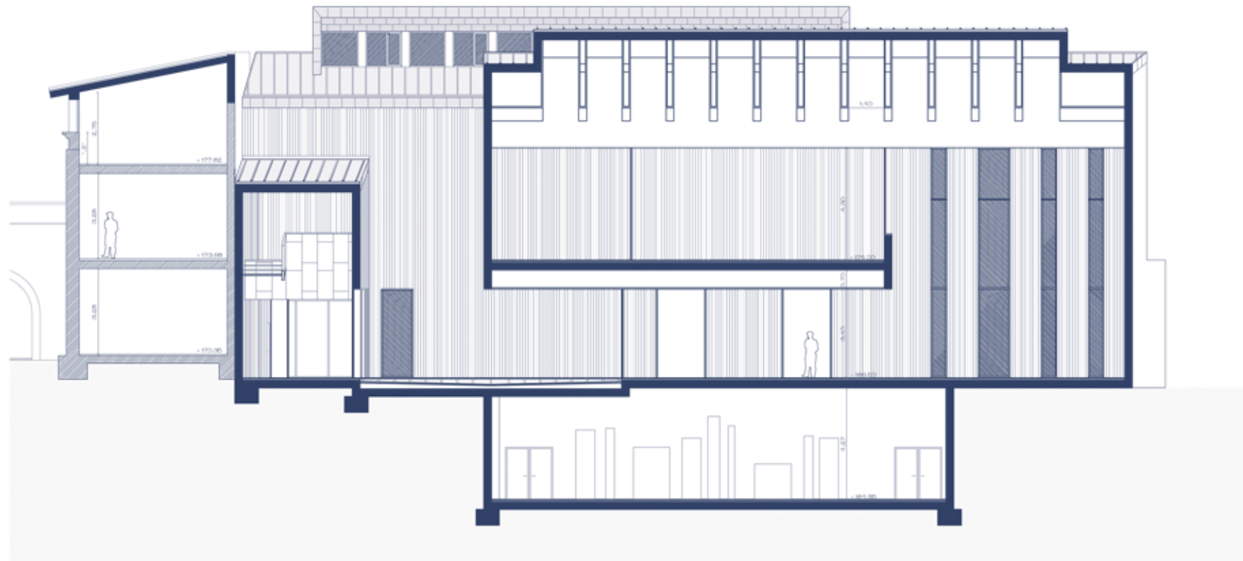
SECCIÓN F F
