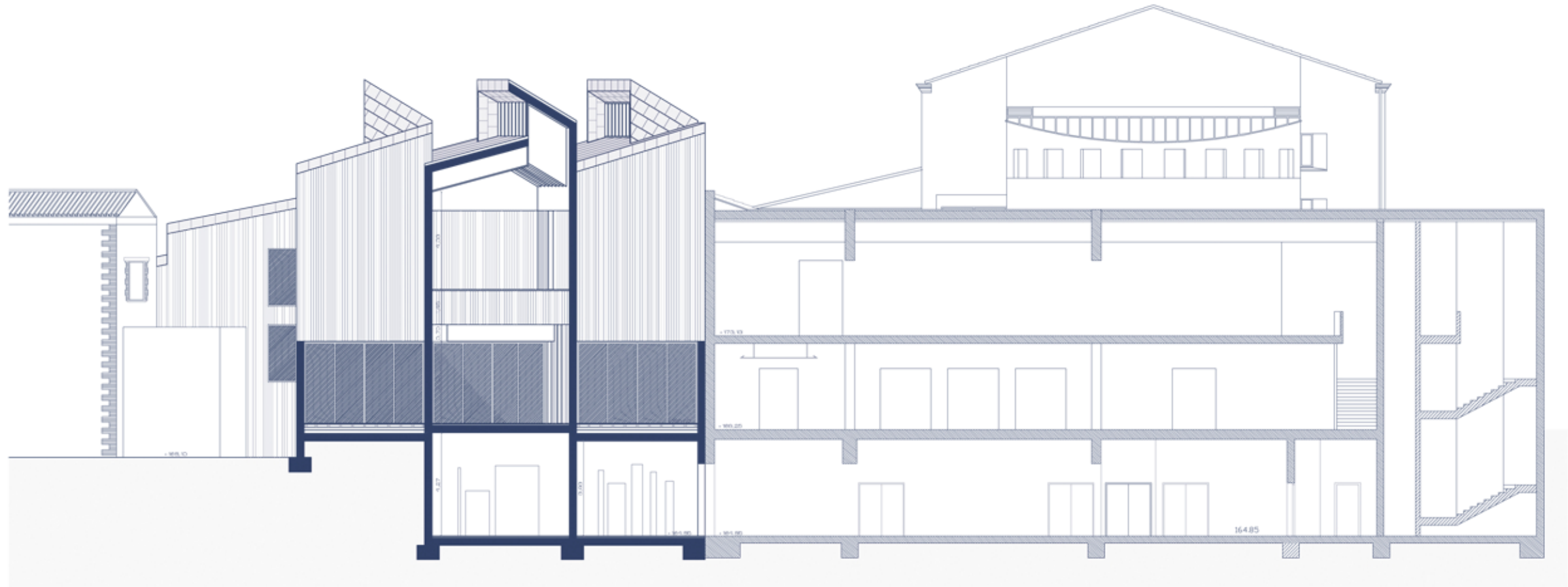
SECCIÓN D D'
