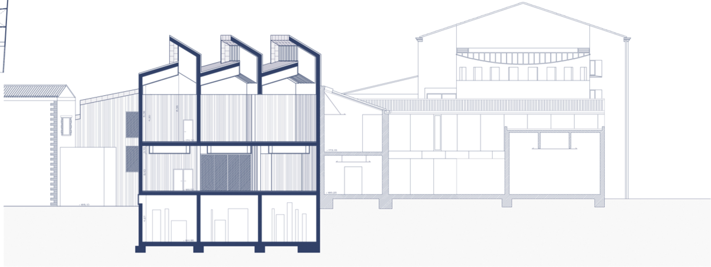
SECCIÓN C C'
