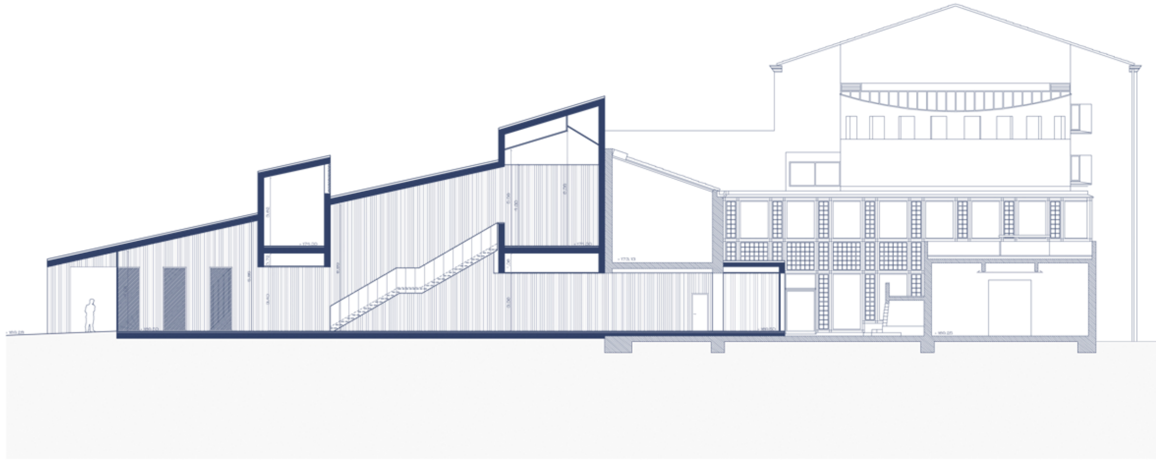
SECCIÓN A A'
