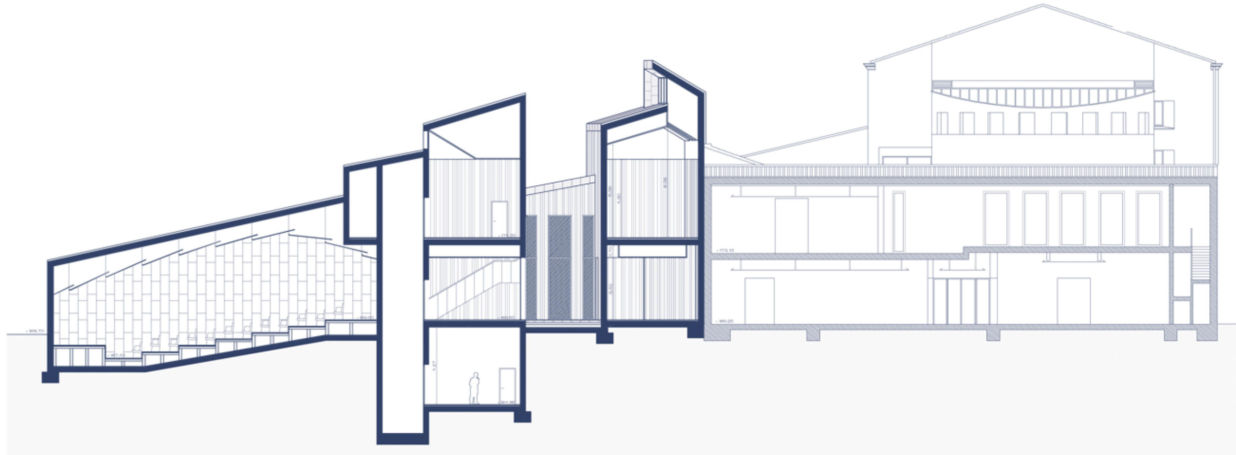
SECCIÓN B B'
