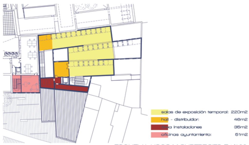
ESQUEMA USOS Y SUPERFICIES E.1/300
