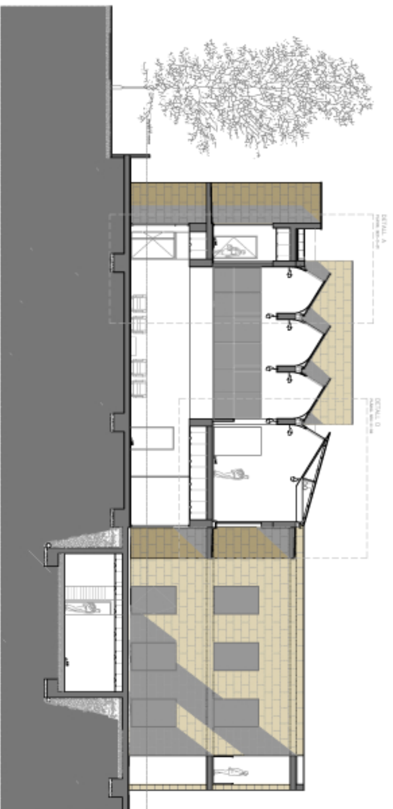
SECCIÓ e--e'
