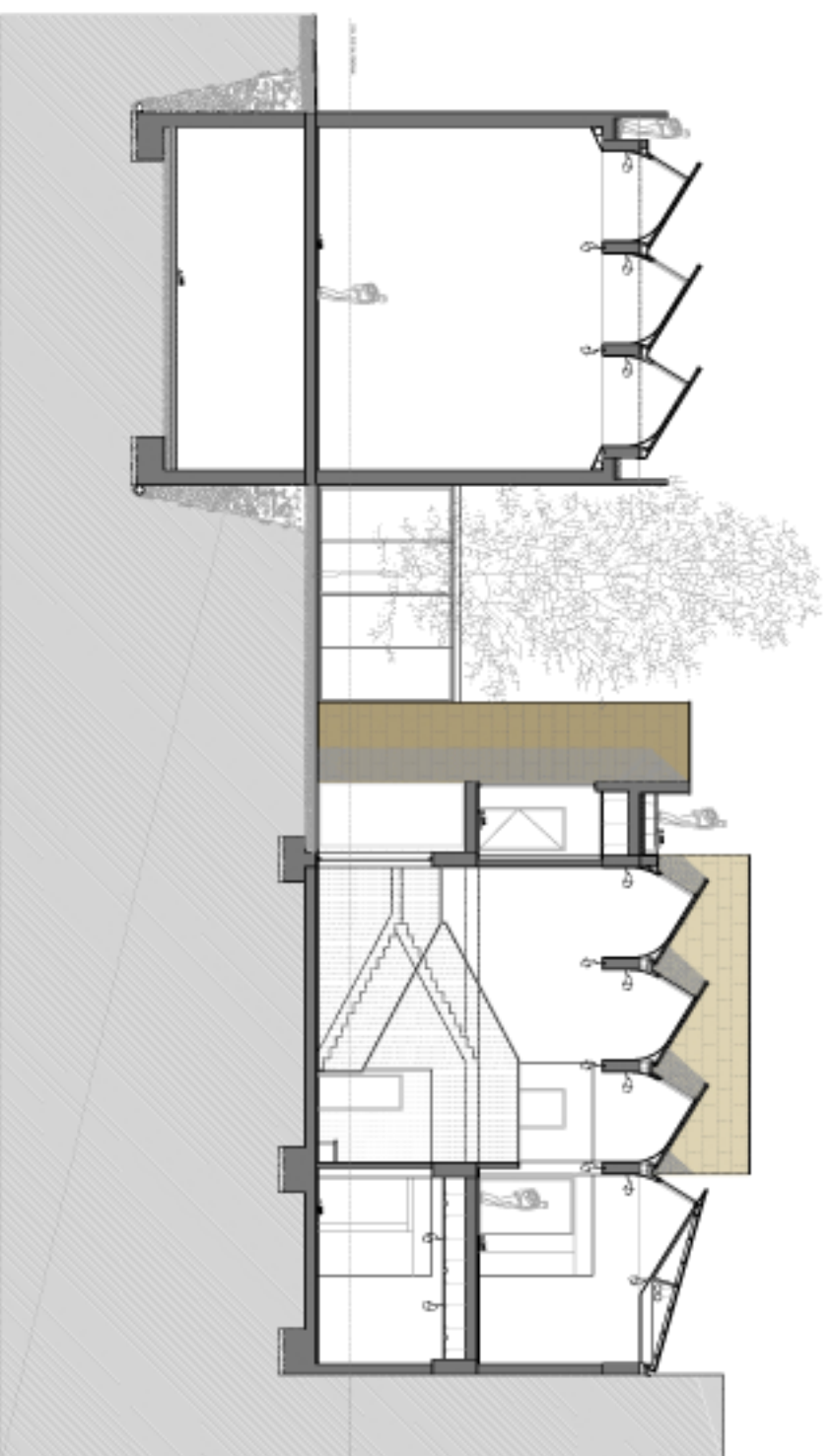
SECCIÓ c-c''
