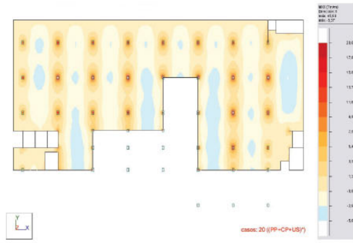
MODELO FORJADOS MOMENTOS MXX
