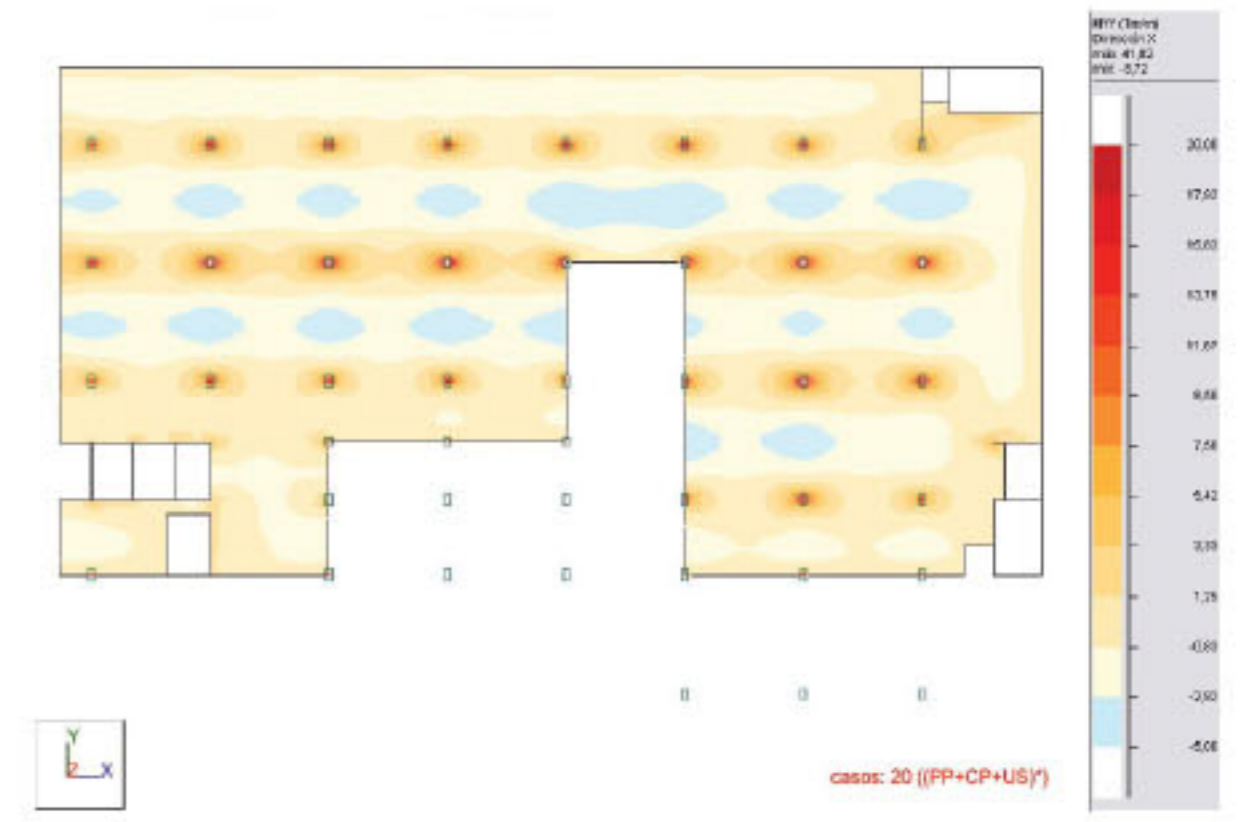
MODELO FORJADOS MOMENTOS MYZ
