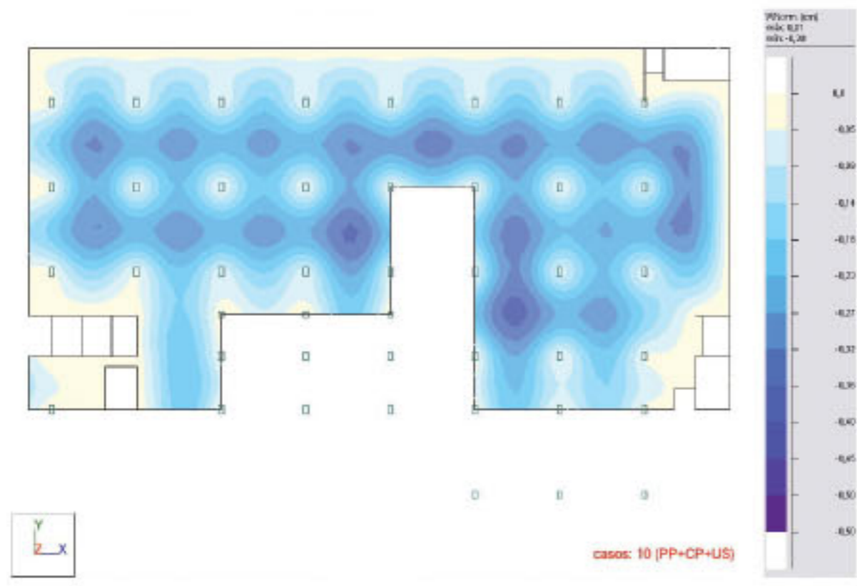
MODELO FORJADOS DEFORMADA
