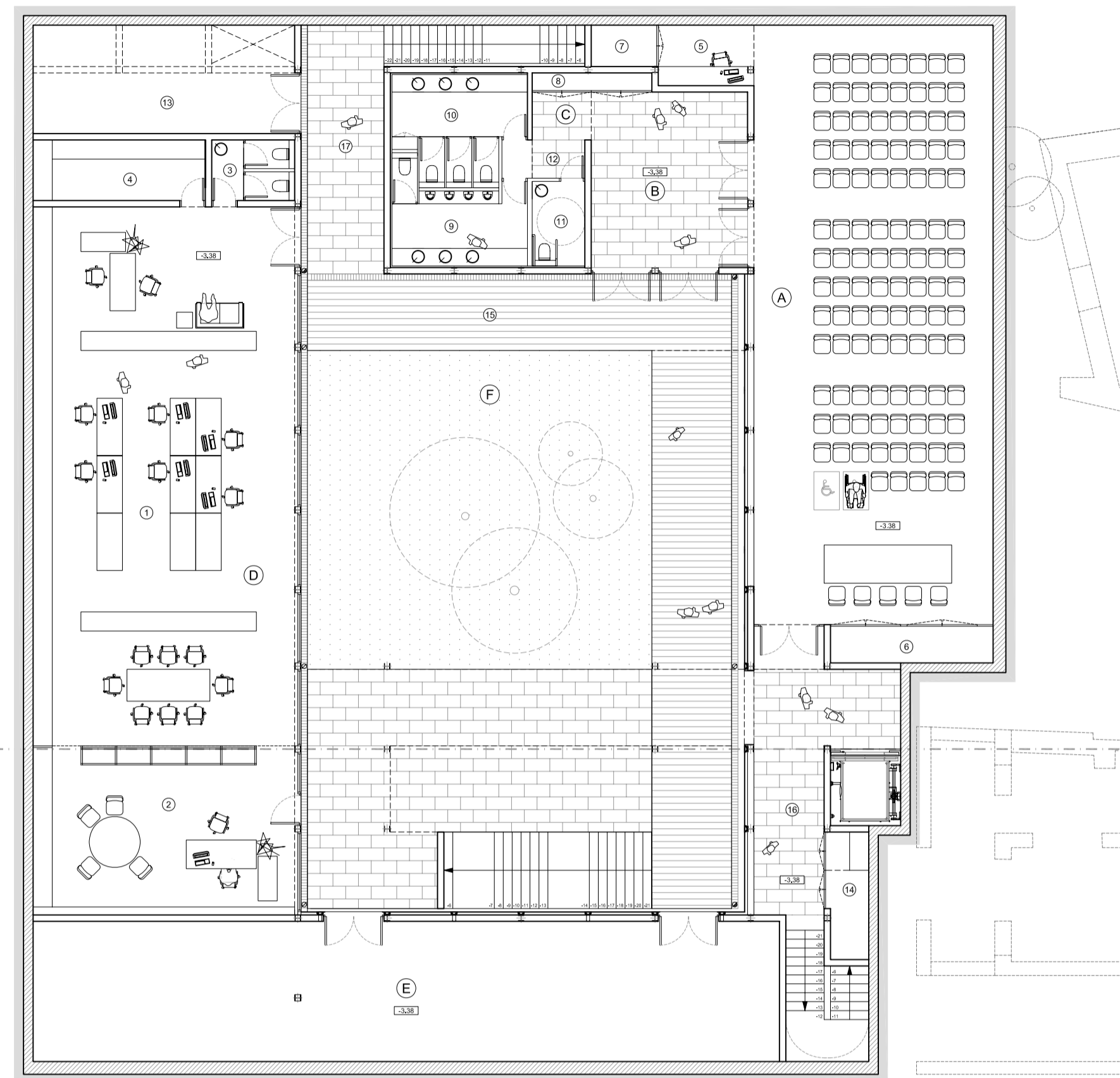
PLANTA SOTERRANI
