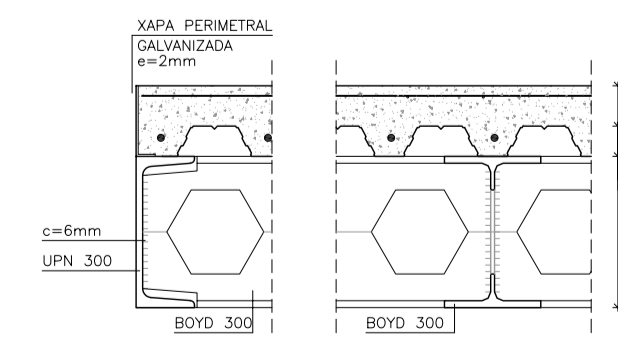
DETALL PERIMETRE FORJAT COL·LABORANT e:1/15
