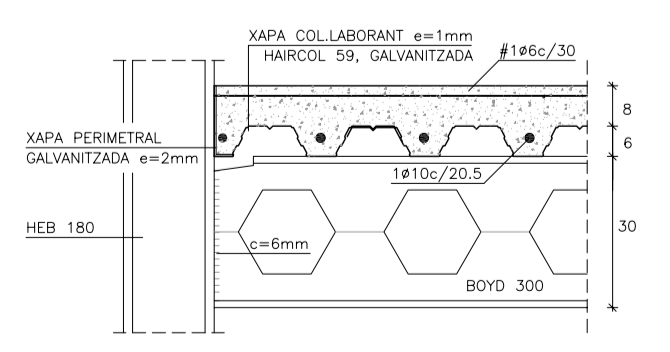
DETALL UNIO TIPUS JASSERA PILAR EN FAÇANA e:1/15
