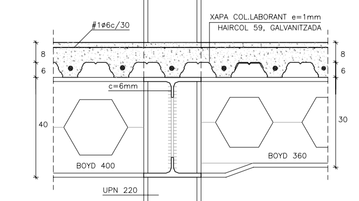
DETALL UNIO ENTRE PERFILS BOYD e:1/15
