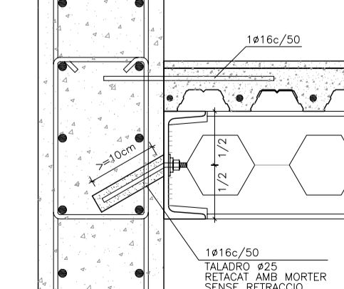
DETALL ANCLATGE PERFIL UPN e:1/15
