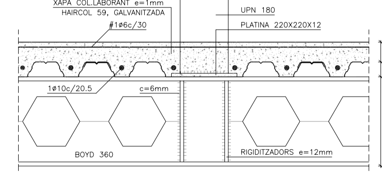
DETALL ESTINTOLAMENT PILAR e:1/15
