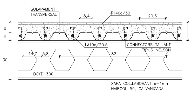
FORJAT COL·LABORANT e:1/15
