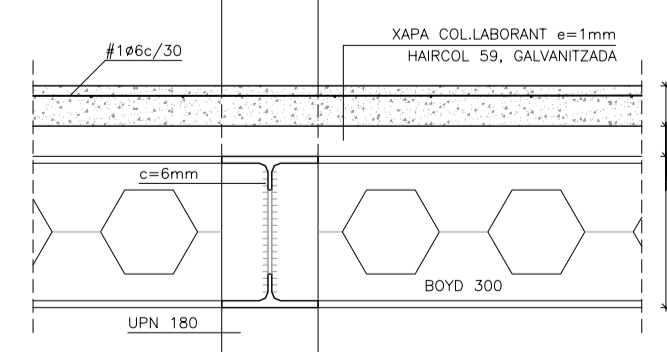
DETALL UNIO TIPUS DE JASSERA I PILARS e:1/15
