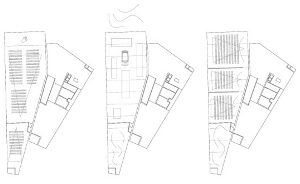
PLANTA ACCESO A SALA GRANDE (+101,70)
