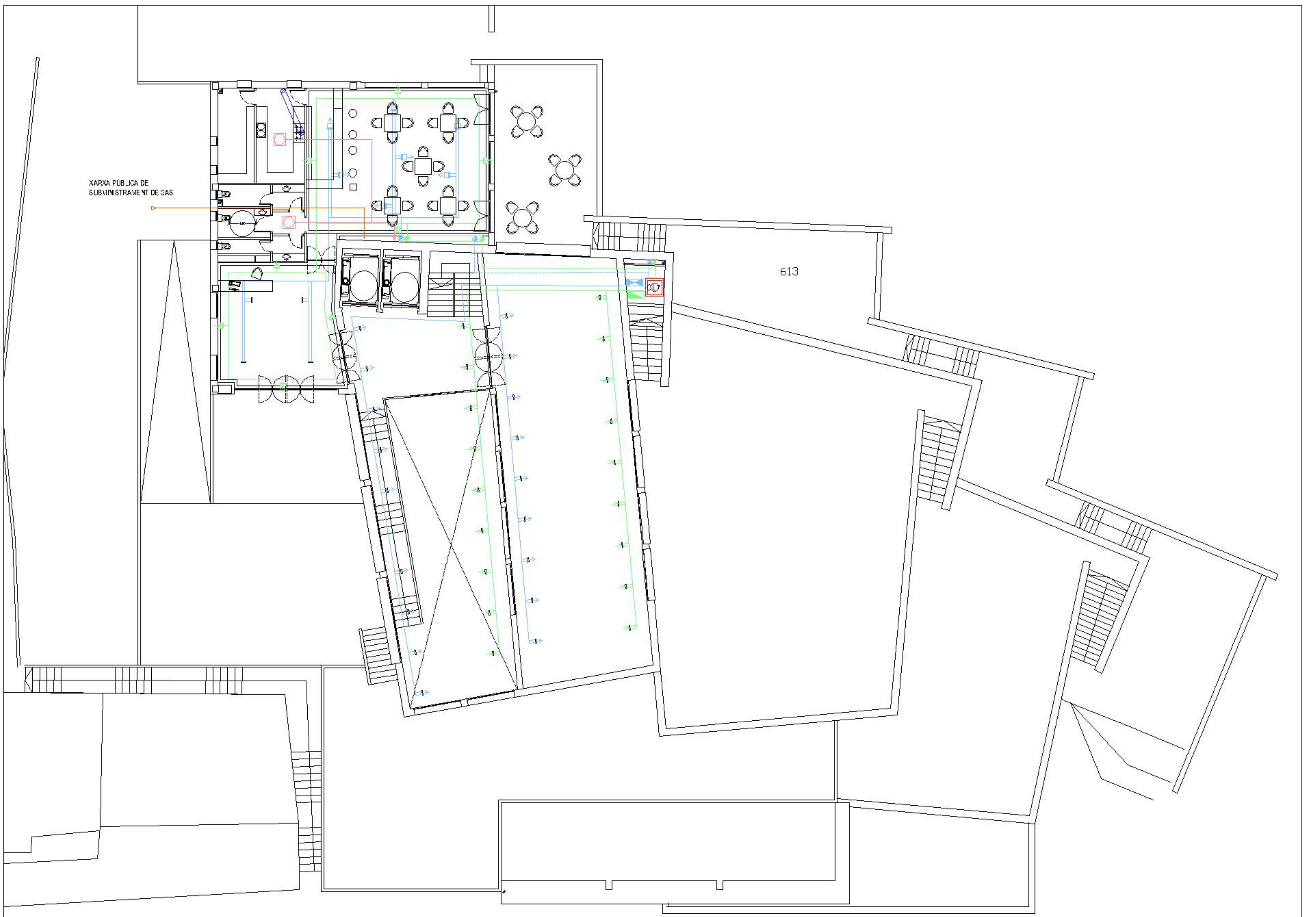
PLANTA COTA 618,8
