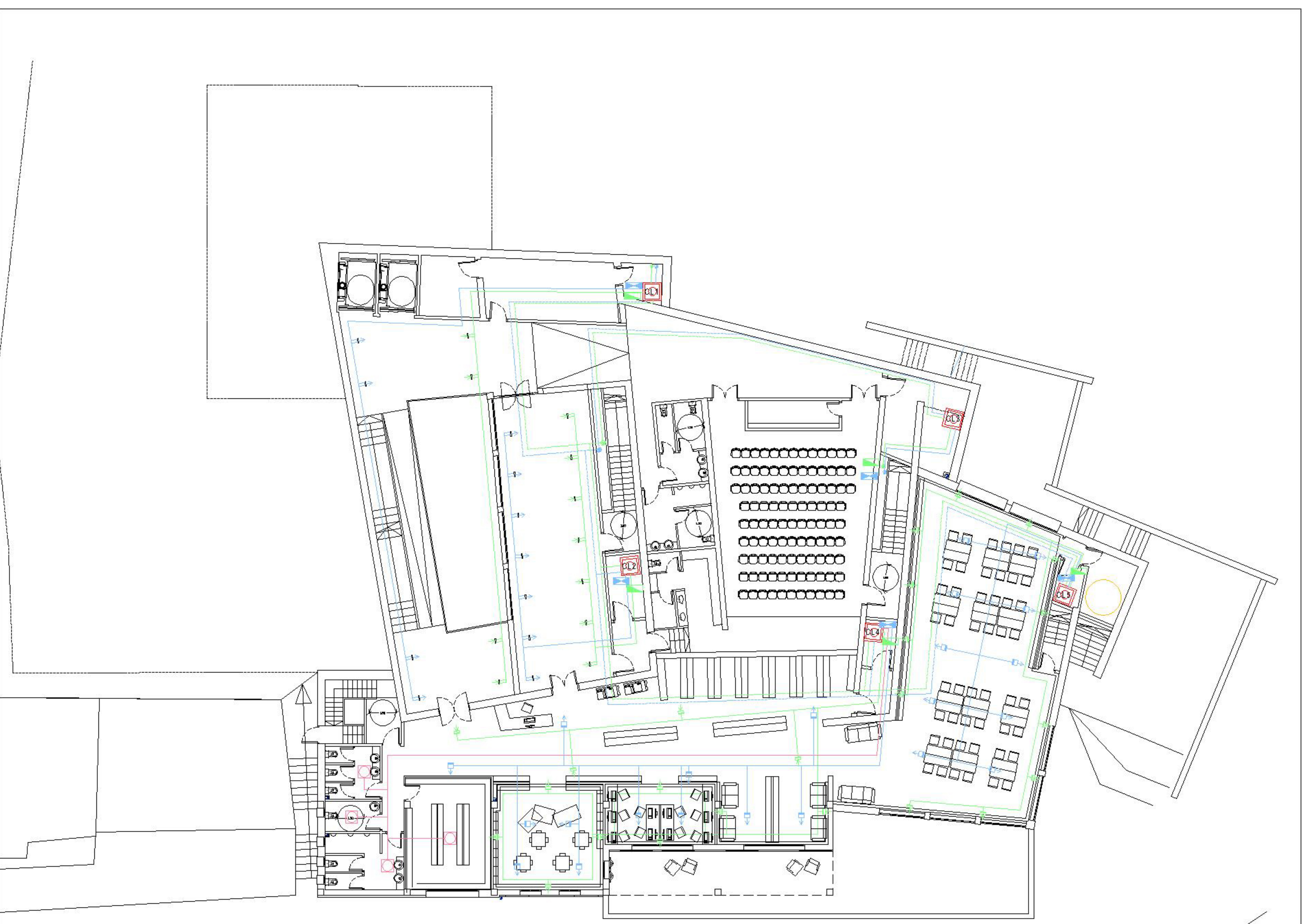
PLANTA COTA 612,2
