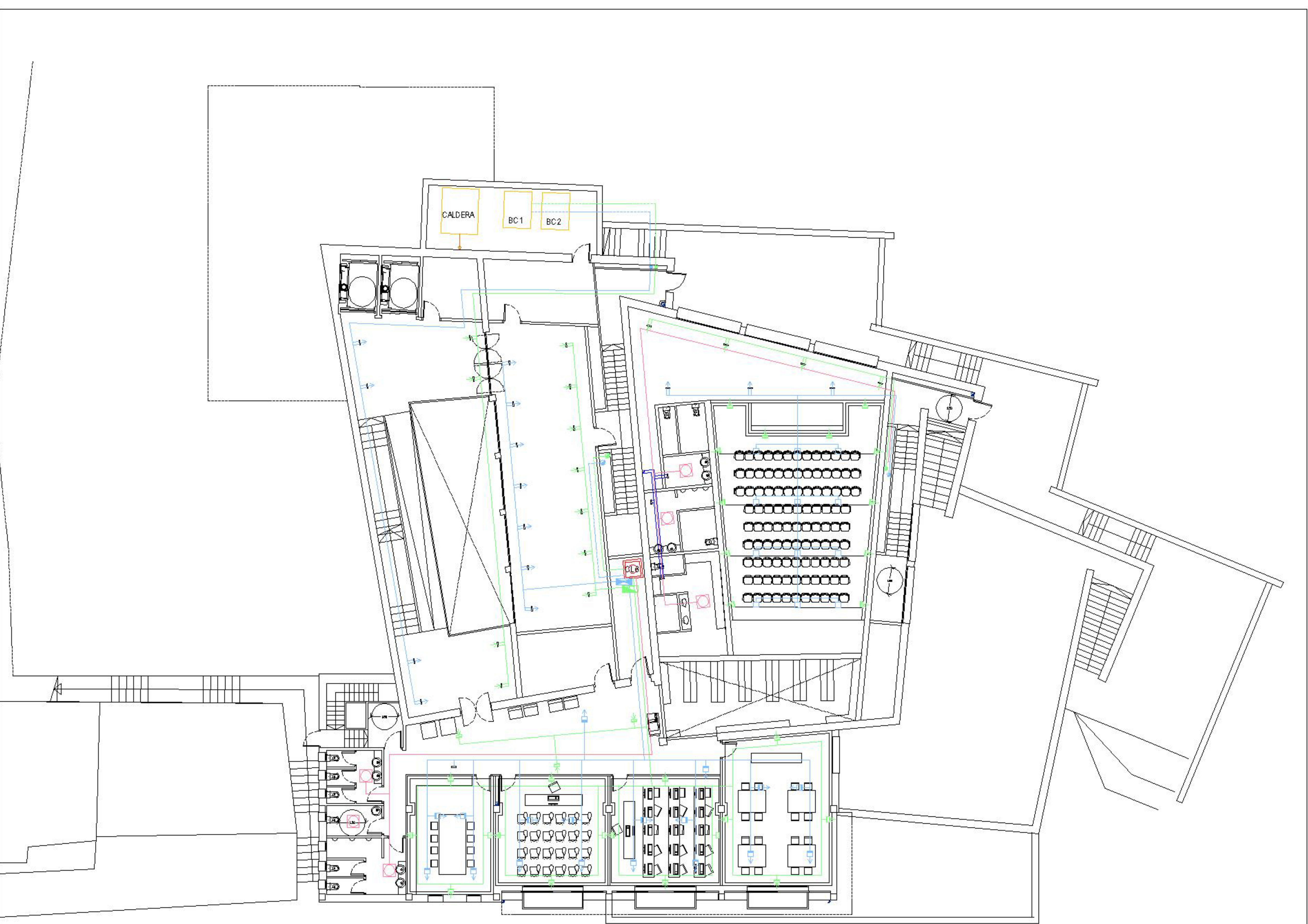
PLANTA COTA 612,2
