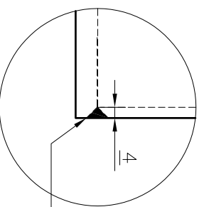
Detall A Escala 1:1
