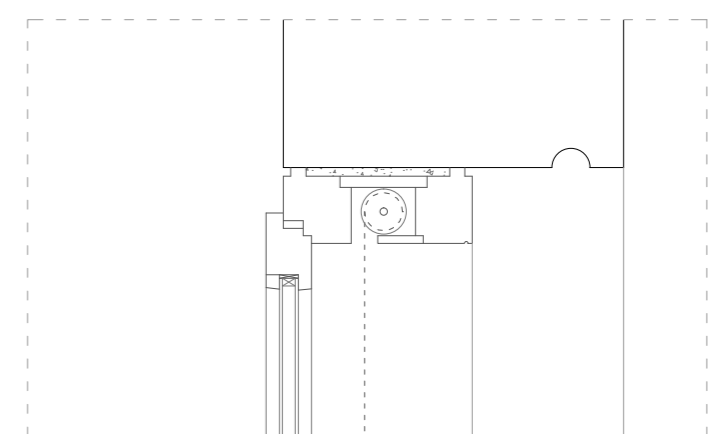
DETALL B
