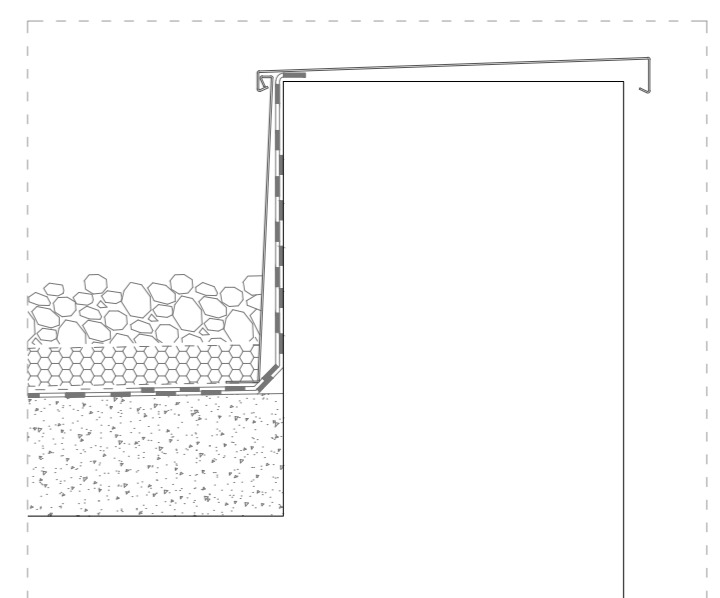
DETALLS FAÇANA ESCALA 1:10
