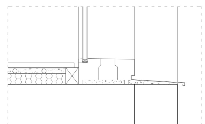
DETALL D
