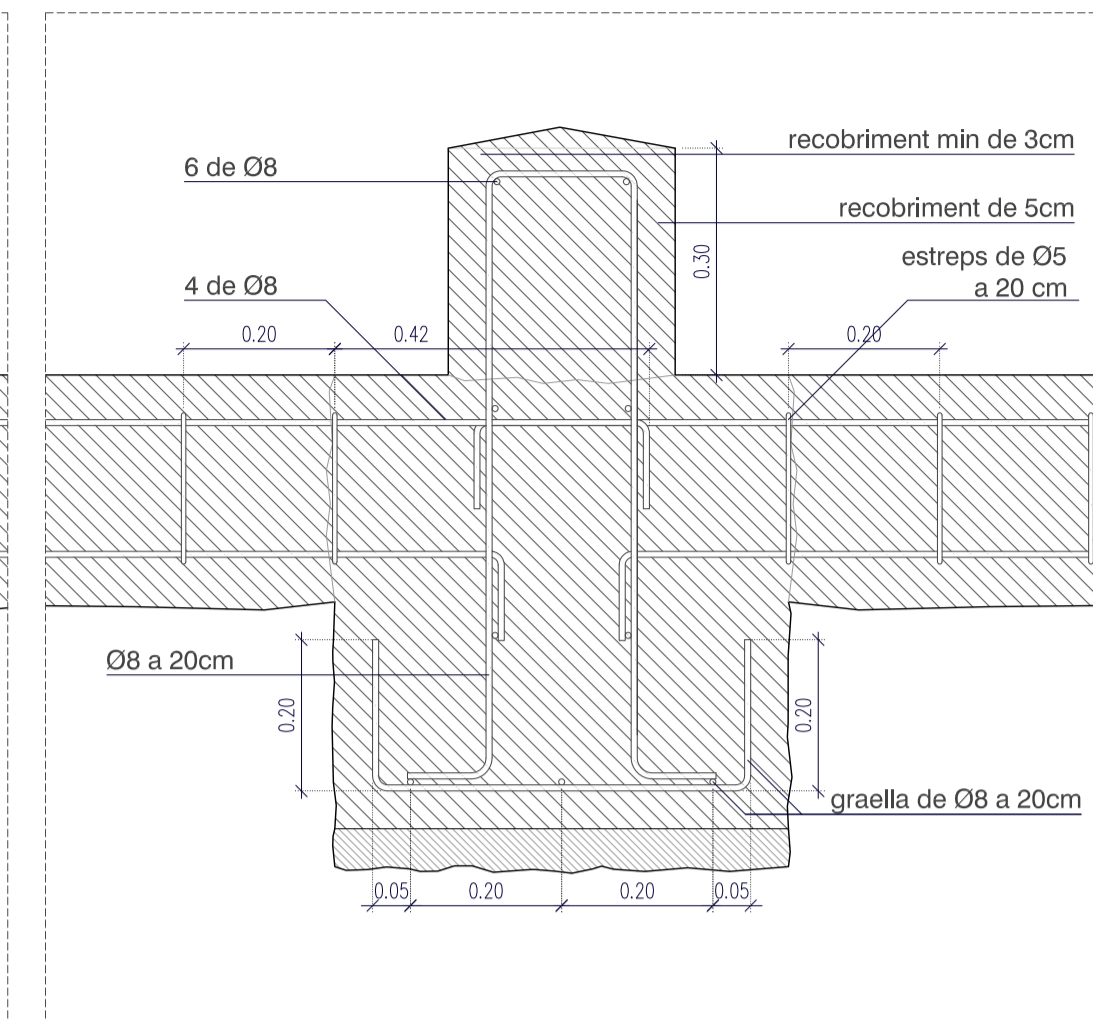
Detall fonamentació D.FO. 02
