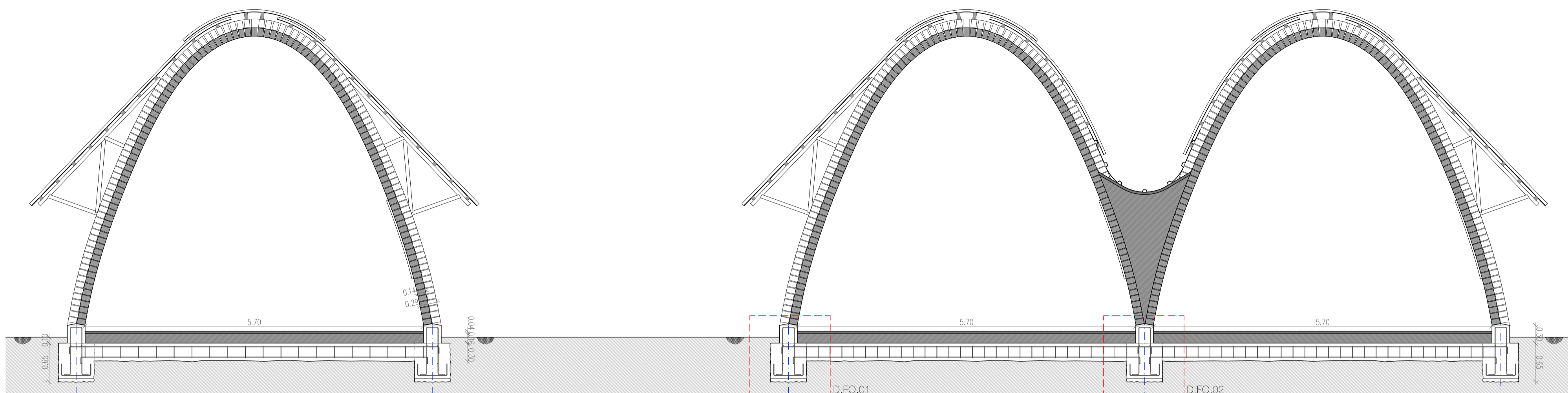
Secció ST.04
