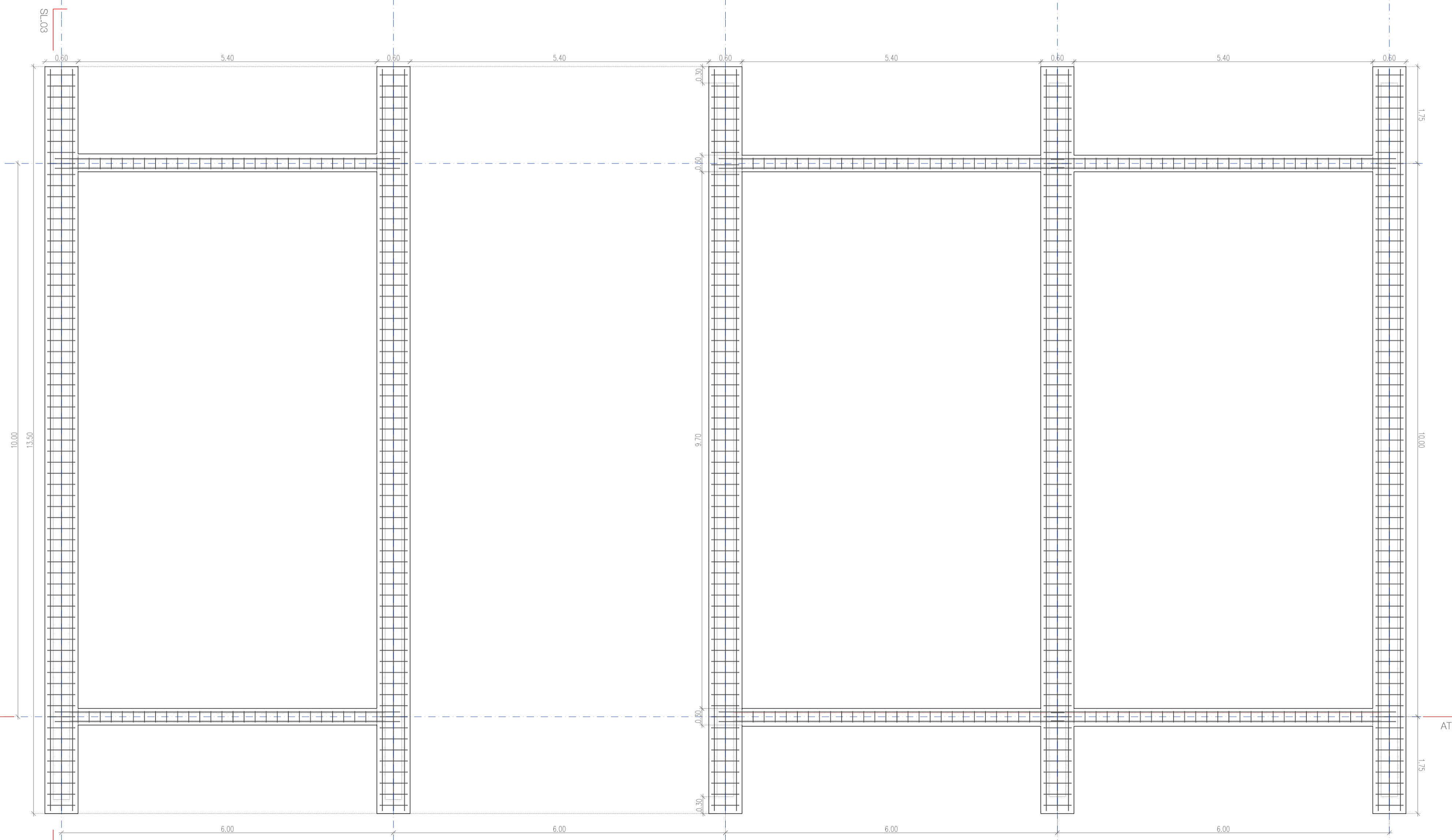
Planta fonaments
