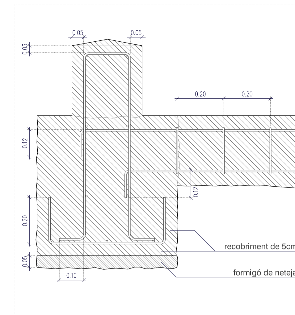
Detall fonamentació D.FO. 01
