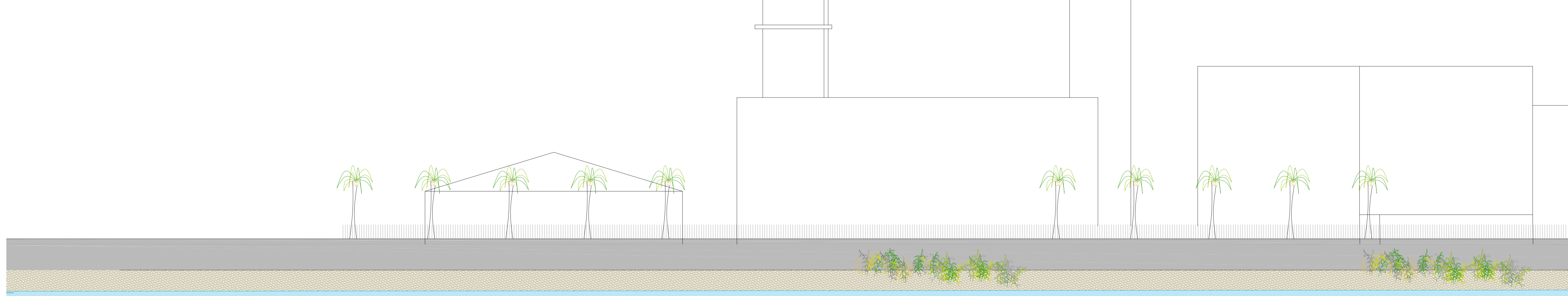
Secció Longitudinal 1
