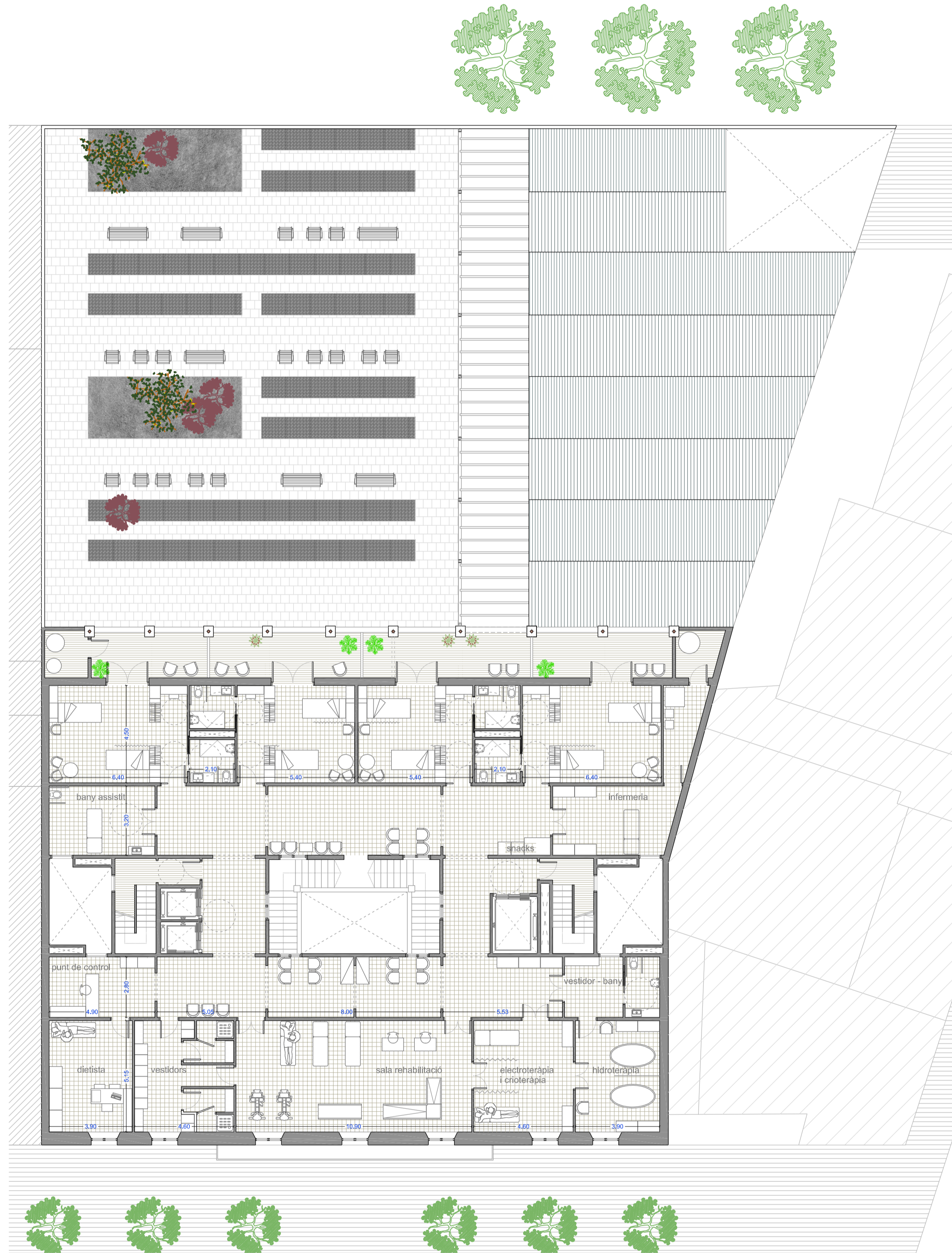
PLANTA PRIMERA _ cota +5'43
