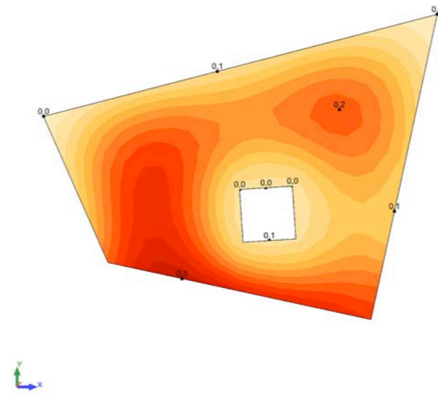
Gràfic de deformacions (Eix Z) (ELS)
