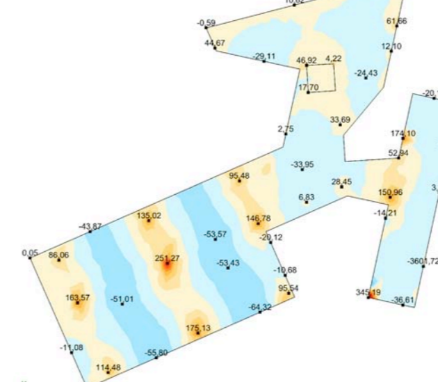
Gràfic de Moments (XX) (ELU)
