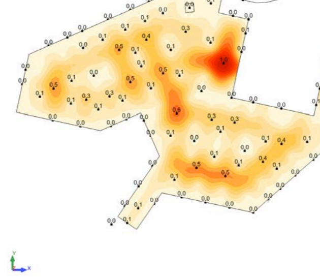
Gràfic de deformacions (Eix Z) (ELS)
