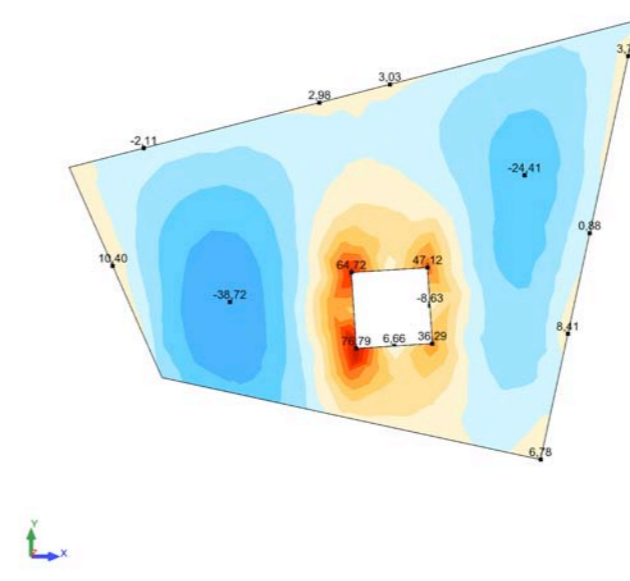
Gràfic de Moments (XX) (ELU)
