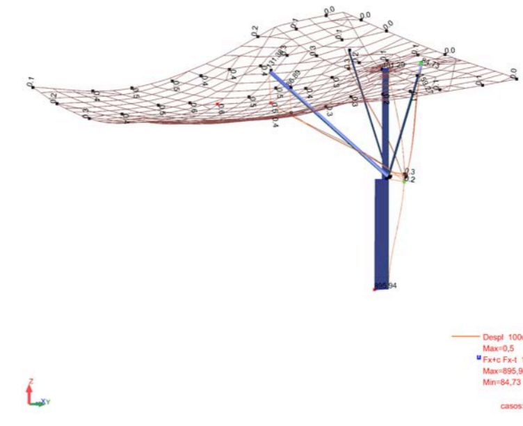
Anàlisi de tensions i deformacions d'un pilar típic
