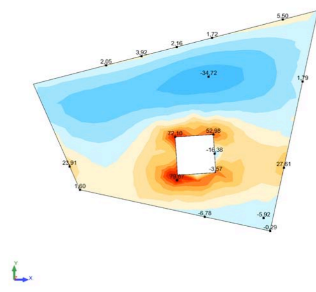
Gràfic de Moments (YY) (ELU)
