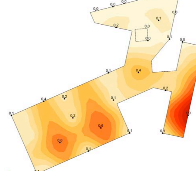
Gràfic de deformacions (Eix Z) (ELS)
