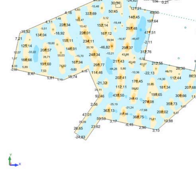
Gràfic de Moments (XX) (ELU)
