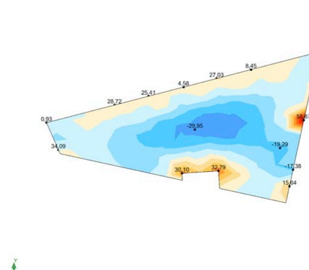
Gràfic de Moments (YY) (ELU)
