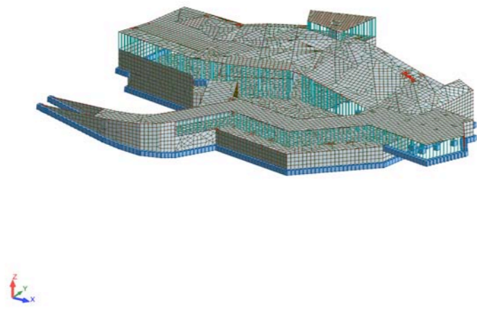
Vista general del model estructural en 3D
