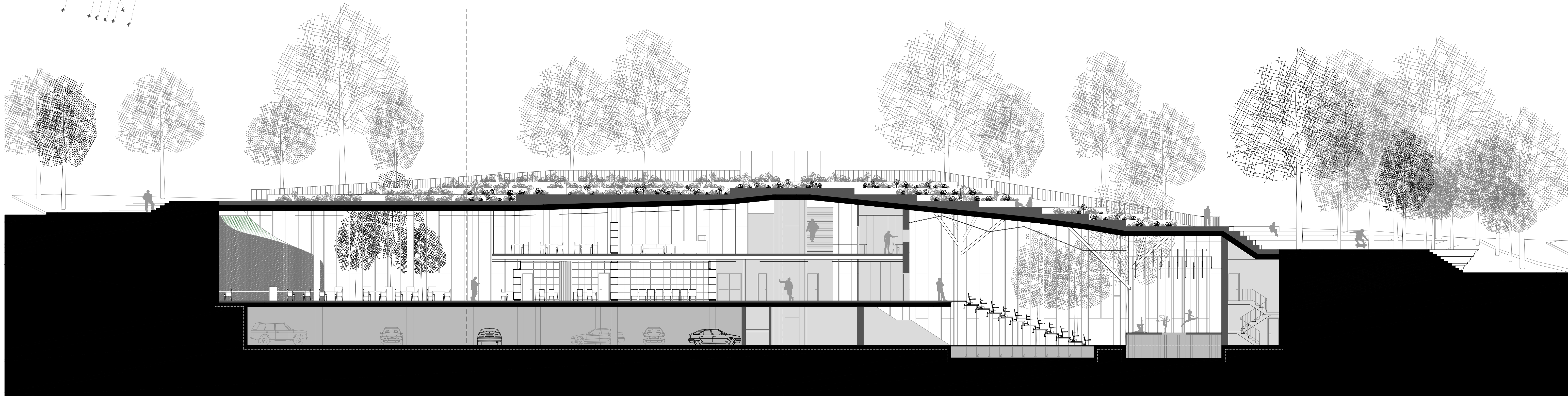
SECCIÓ LONGITUDINAL 01
