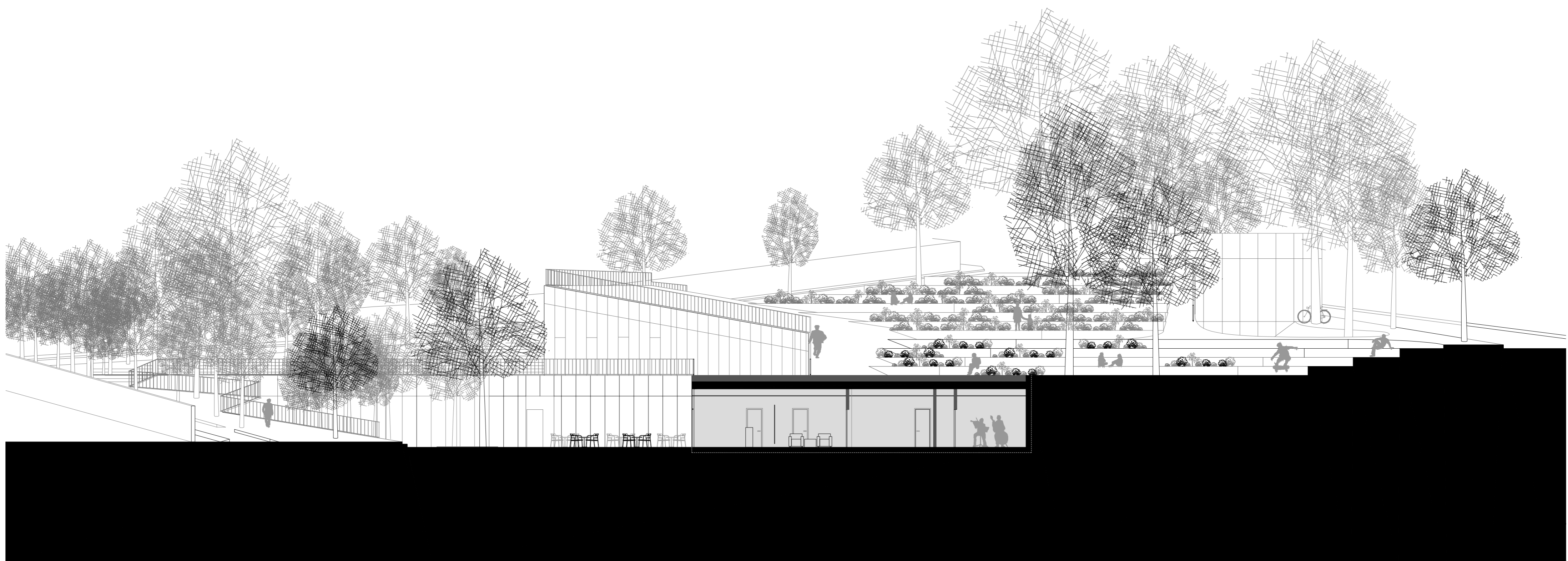
SECCIÓ TRANSVERSAL 07
