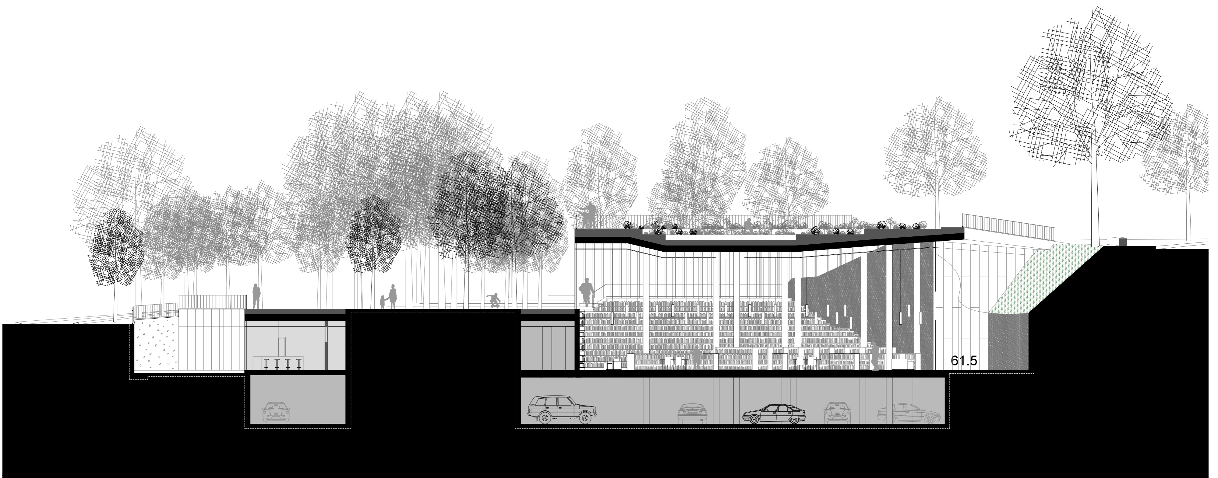
SECCIÓ TRANSVERSAL 02
