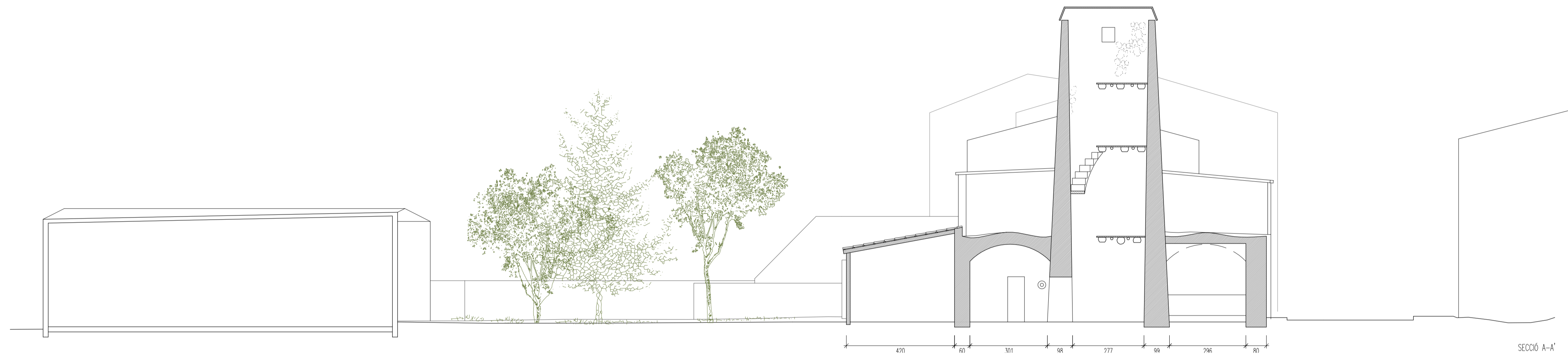
SECCÓ A-A'
