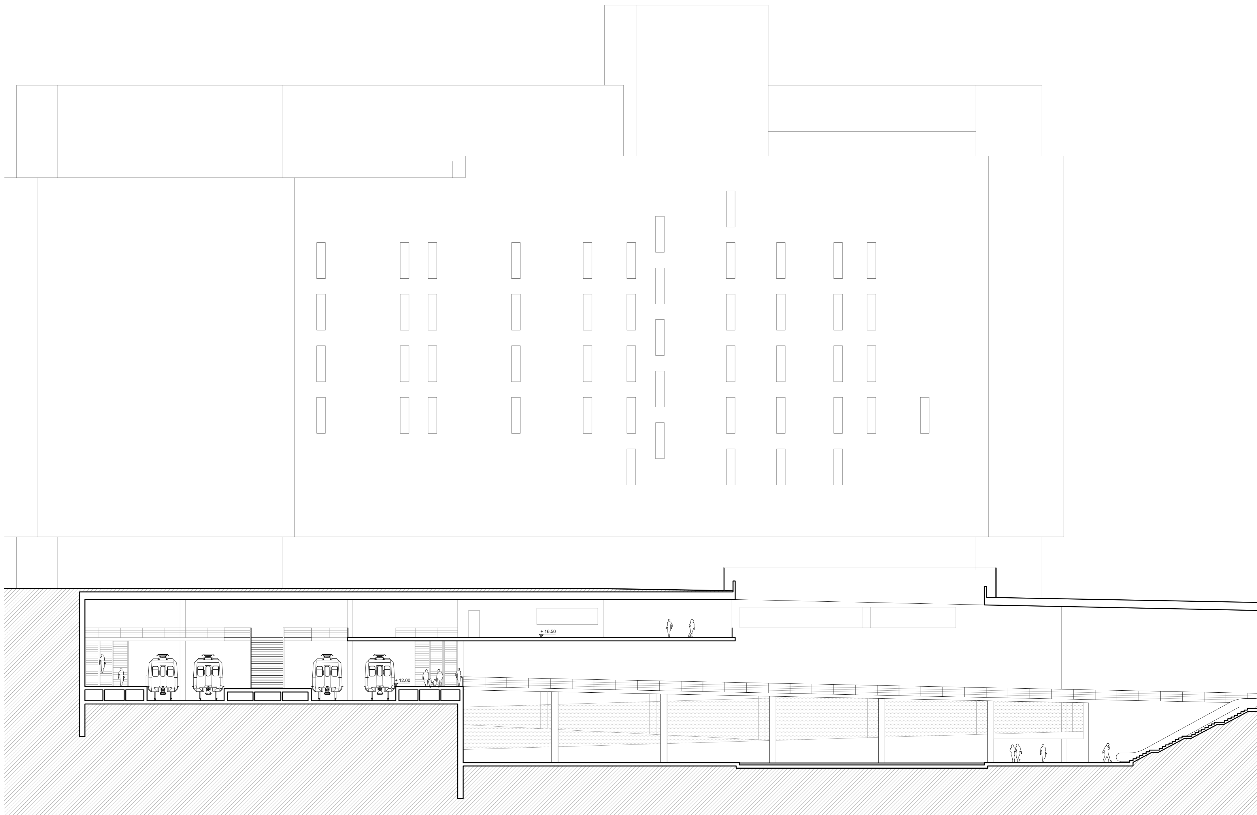
secció G-G'
