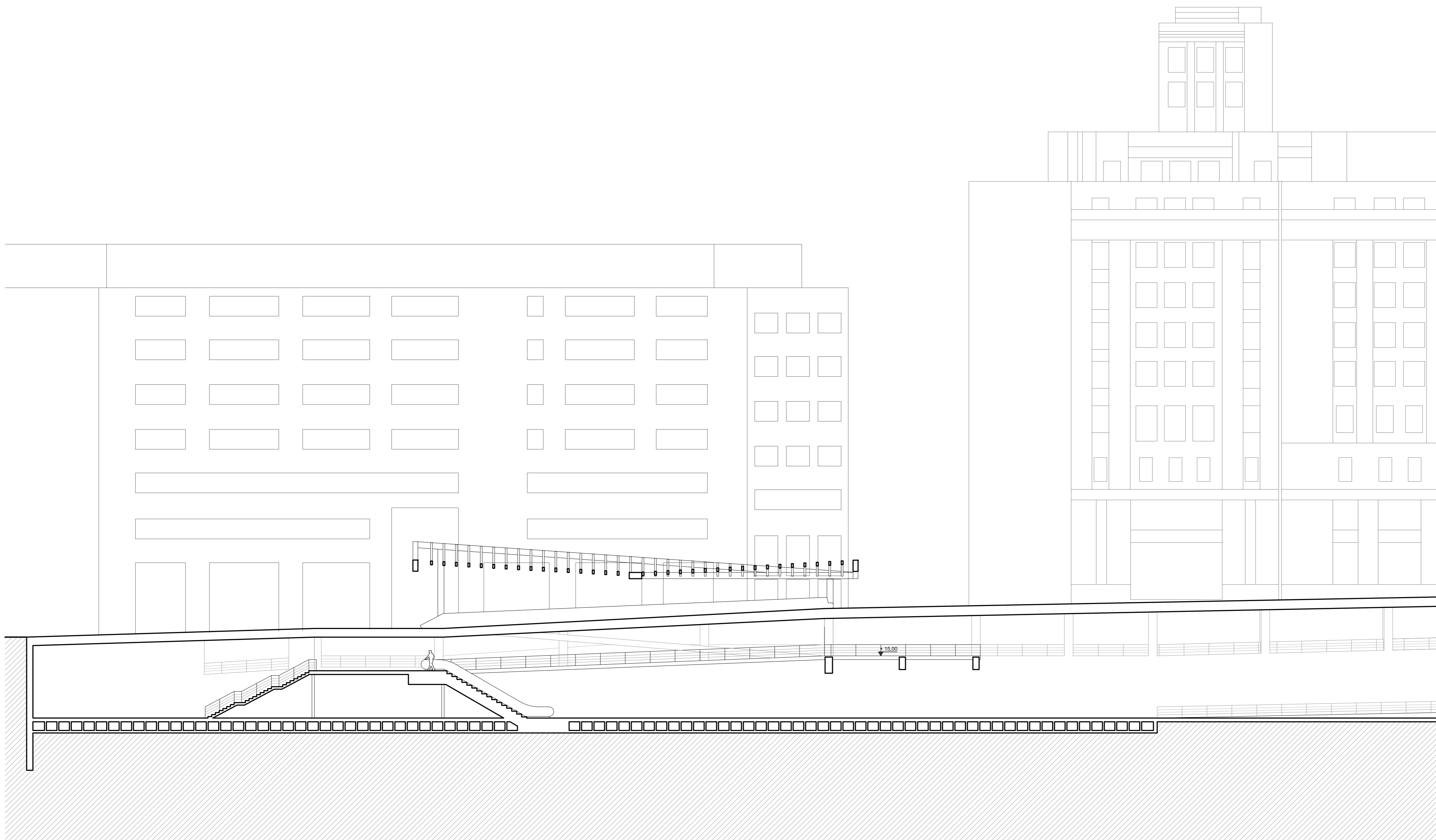
secció H-H'
