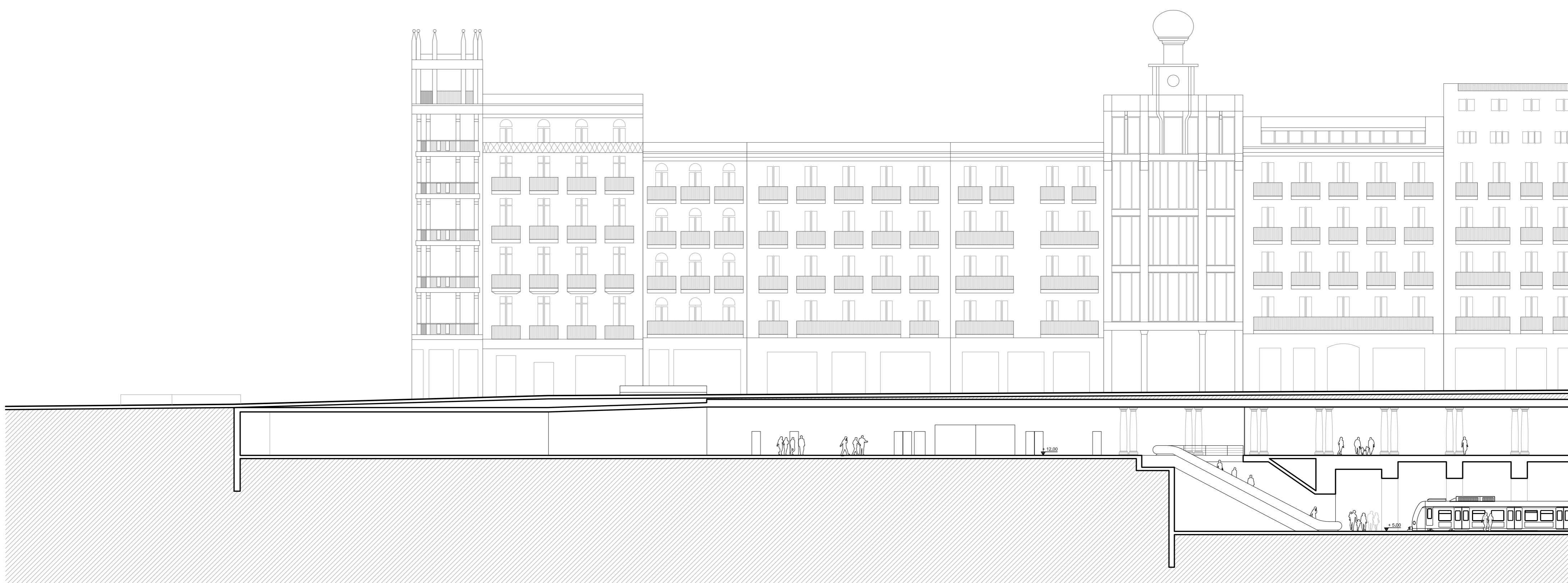
secció F-F'
