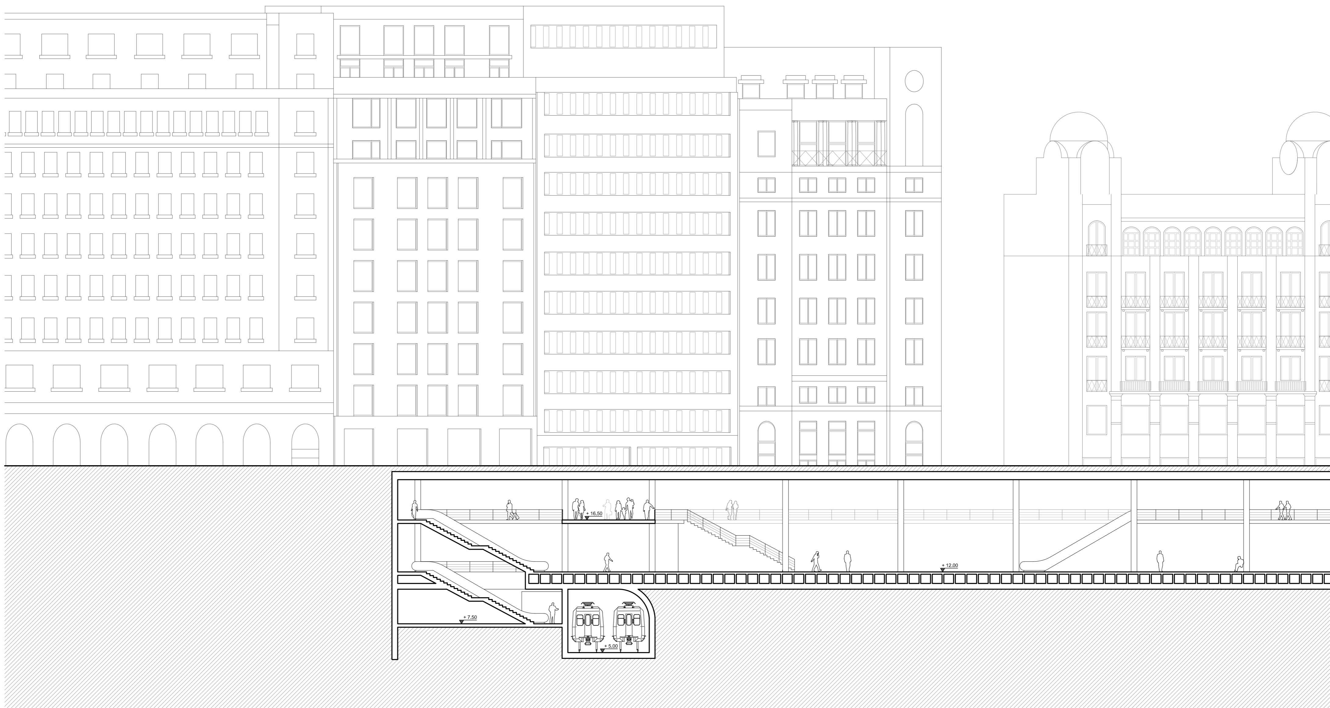
secció A-A'
