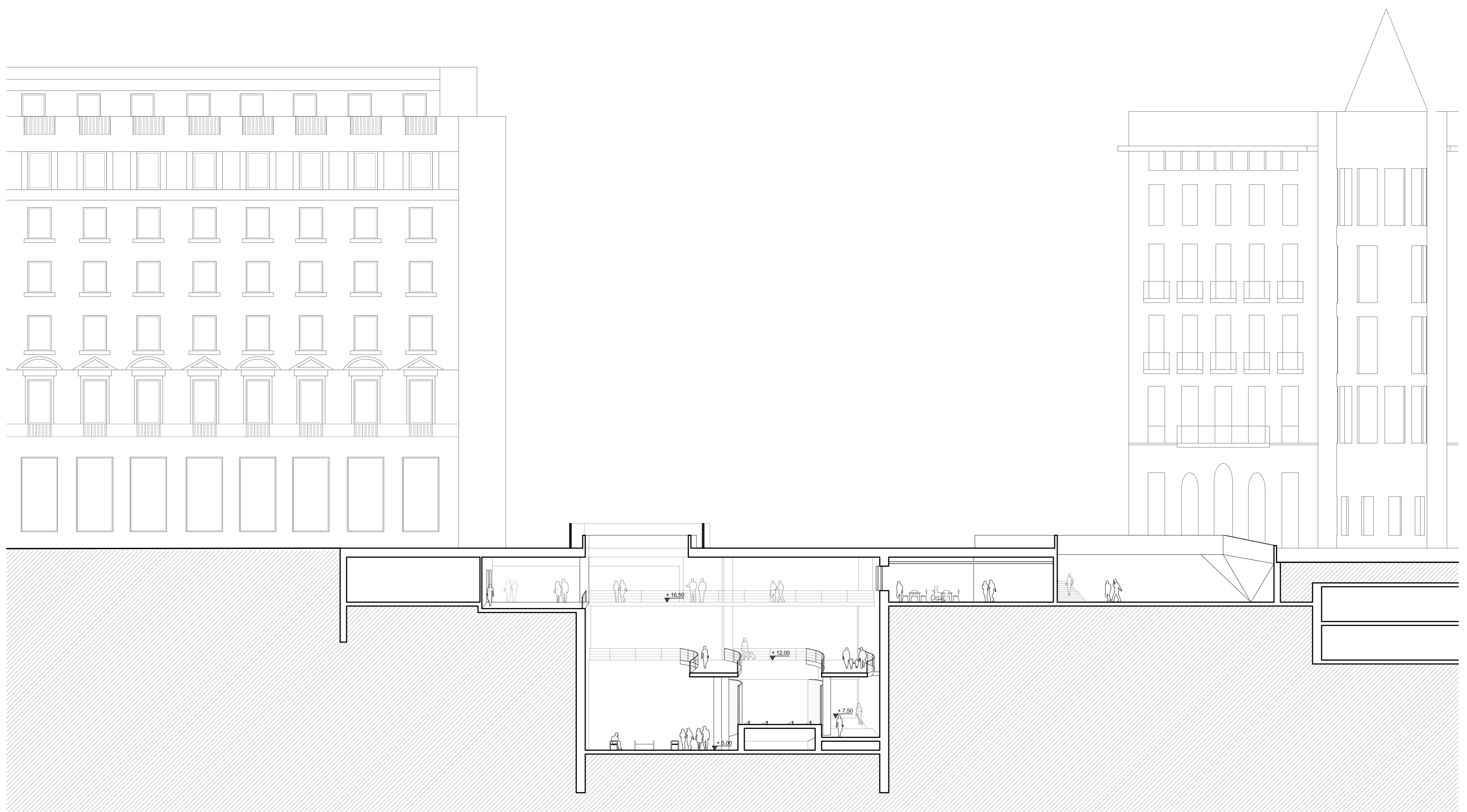
secció C-C'
