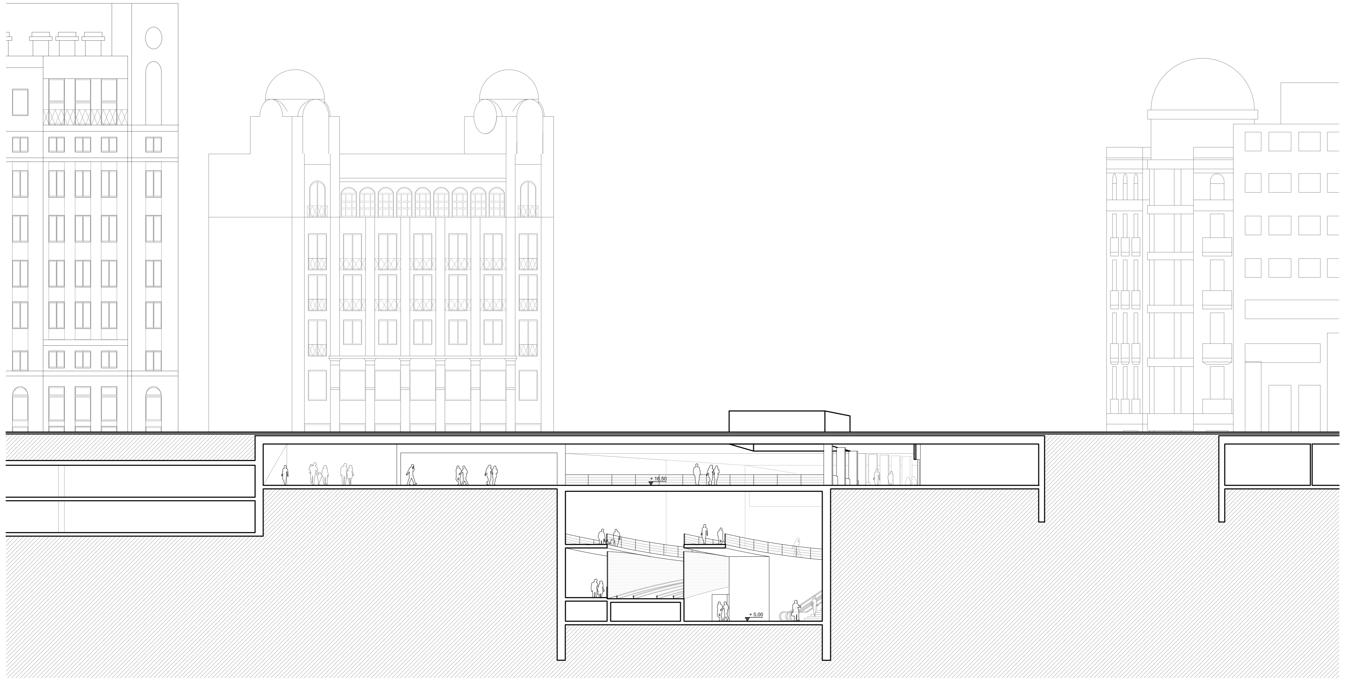
secció B-B'
