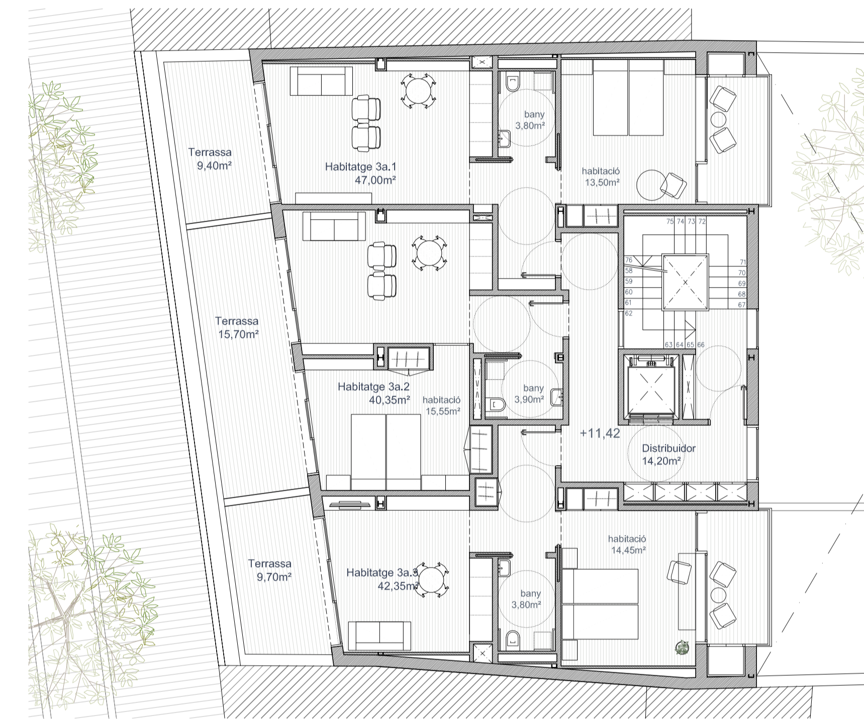
exemple habitages d'ús doble e:1/100
