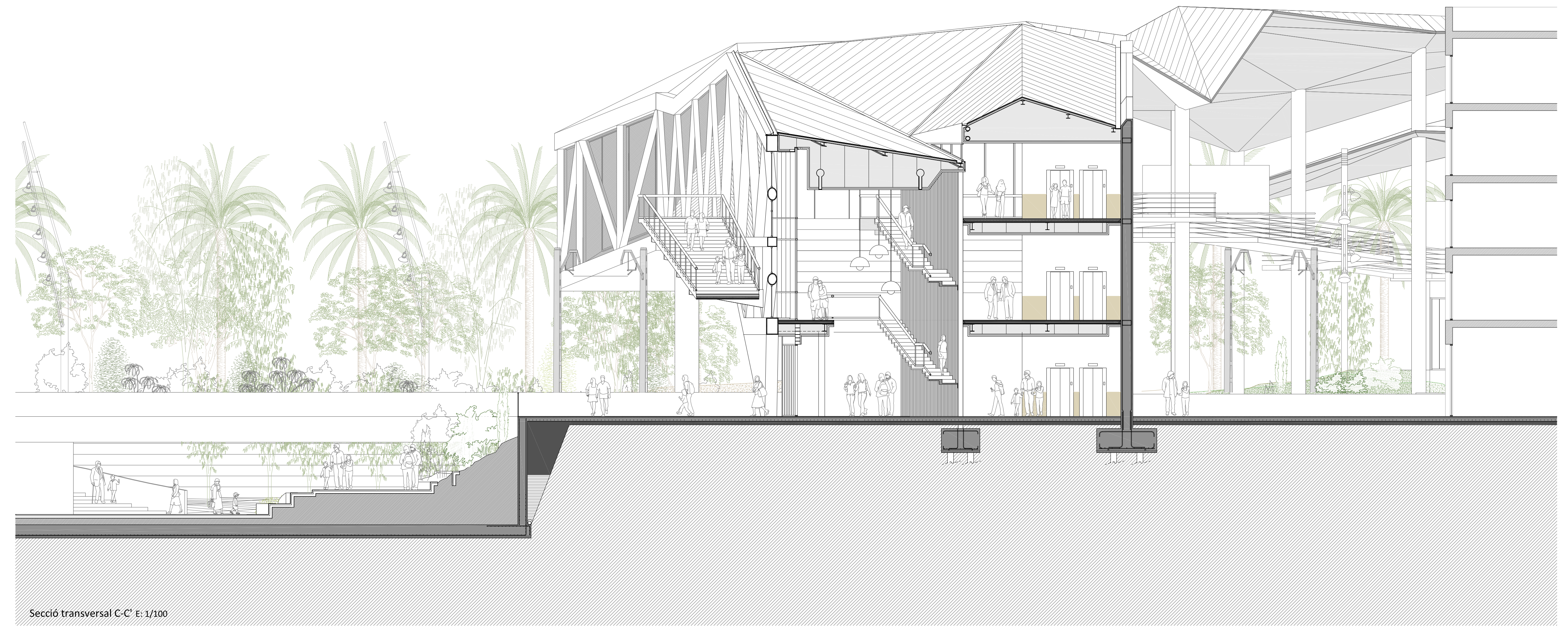
Secció transversal C-C' E: 1/100
