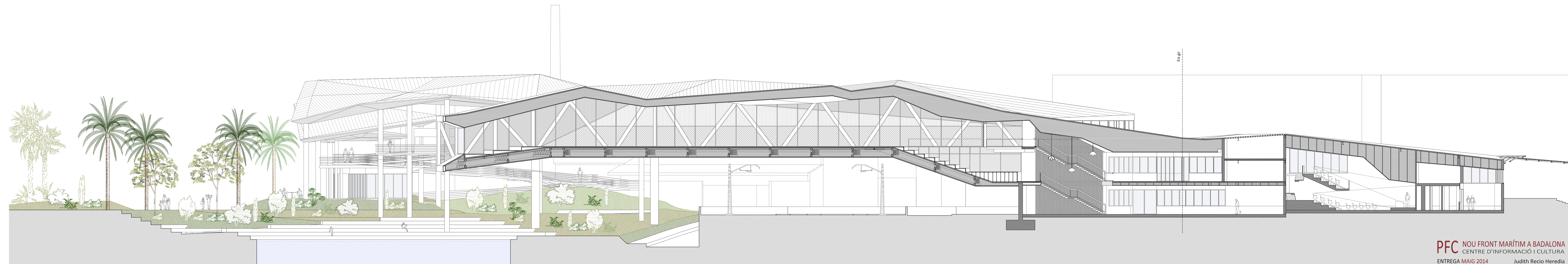
Secció longitudinal E-E' E: 1/150
