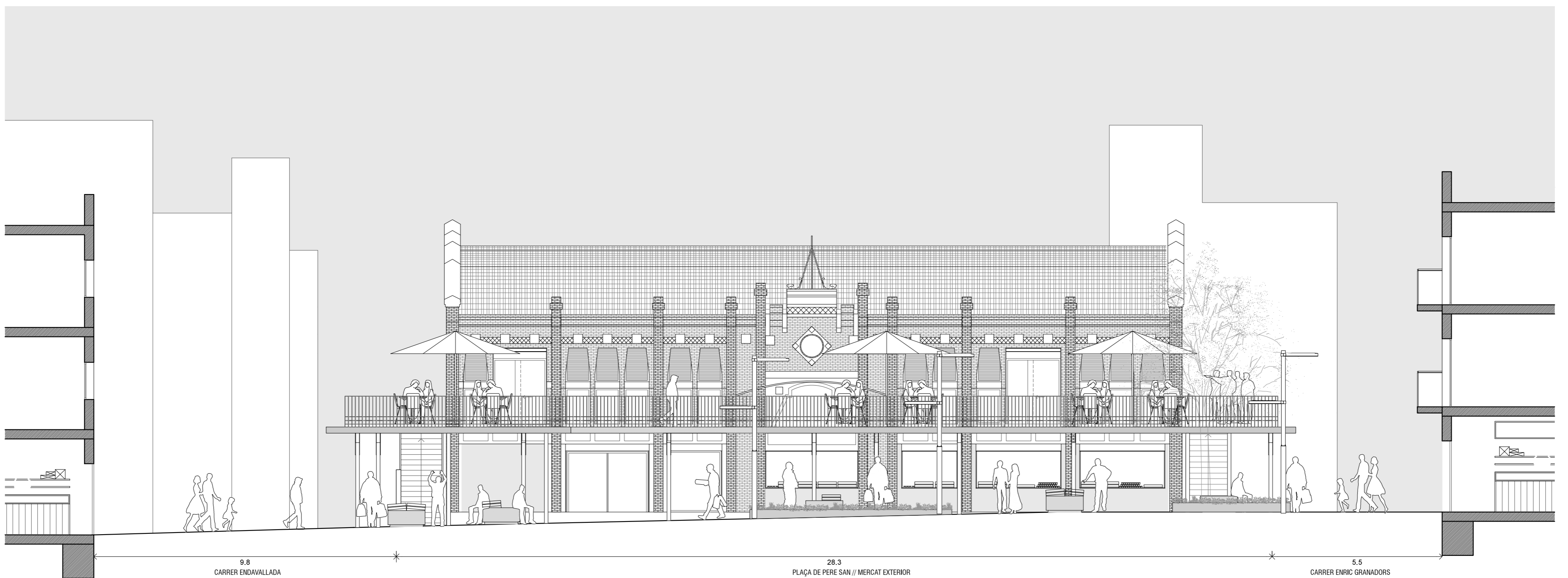
Alçat C plaça e1/100
