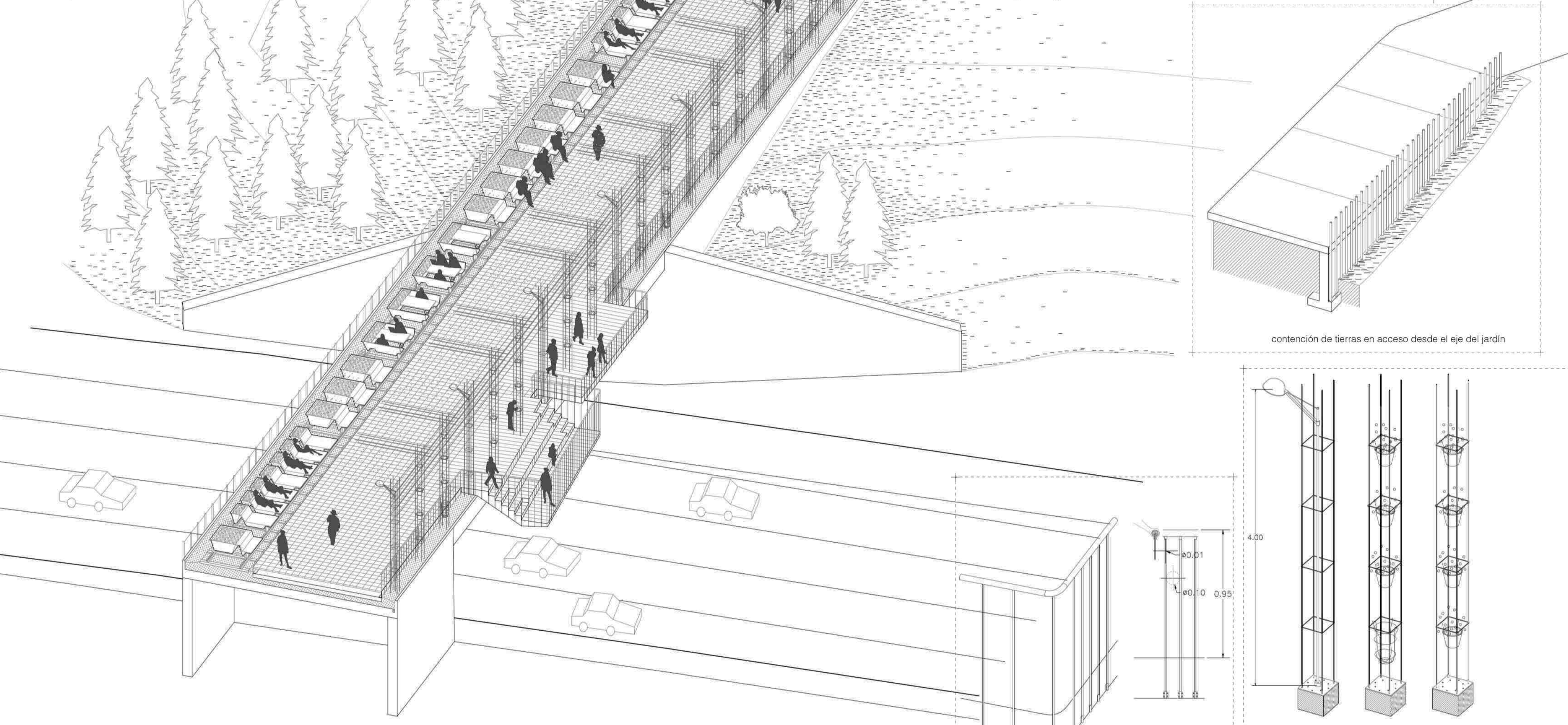
detalle barandilla 1/20
