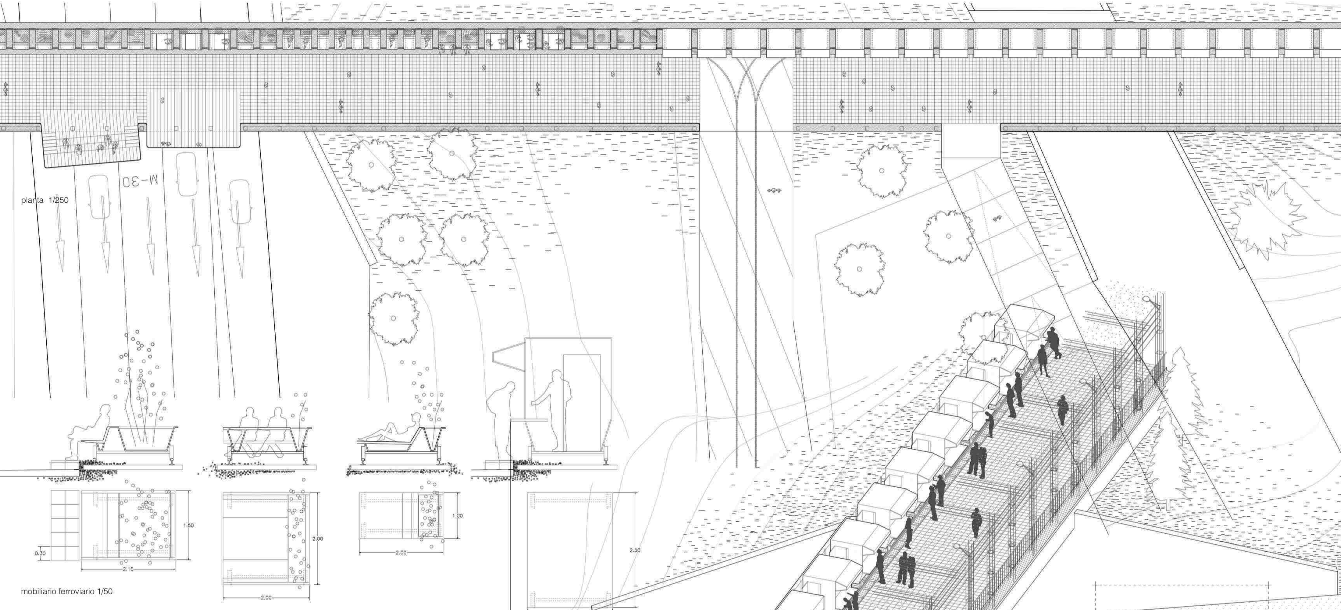
alzado oeste 1/200
