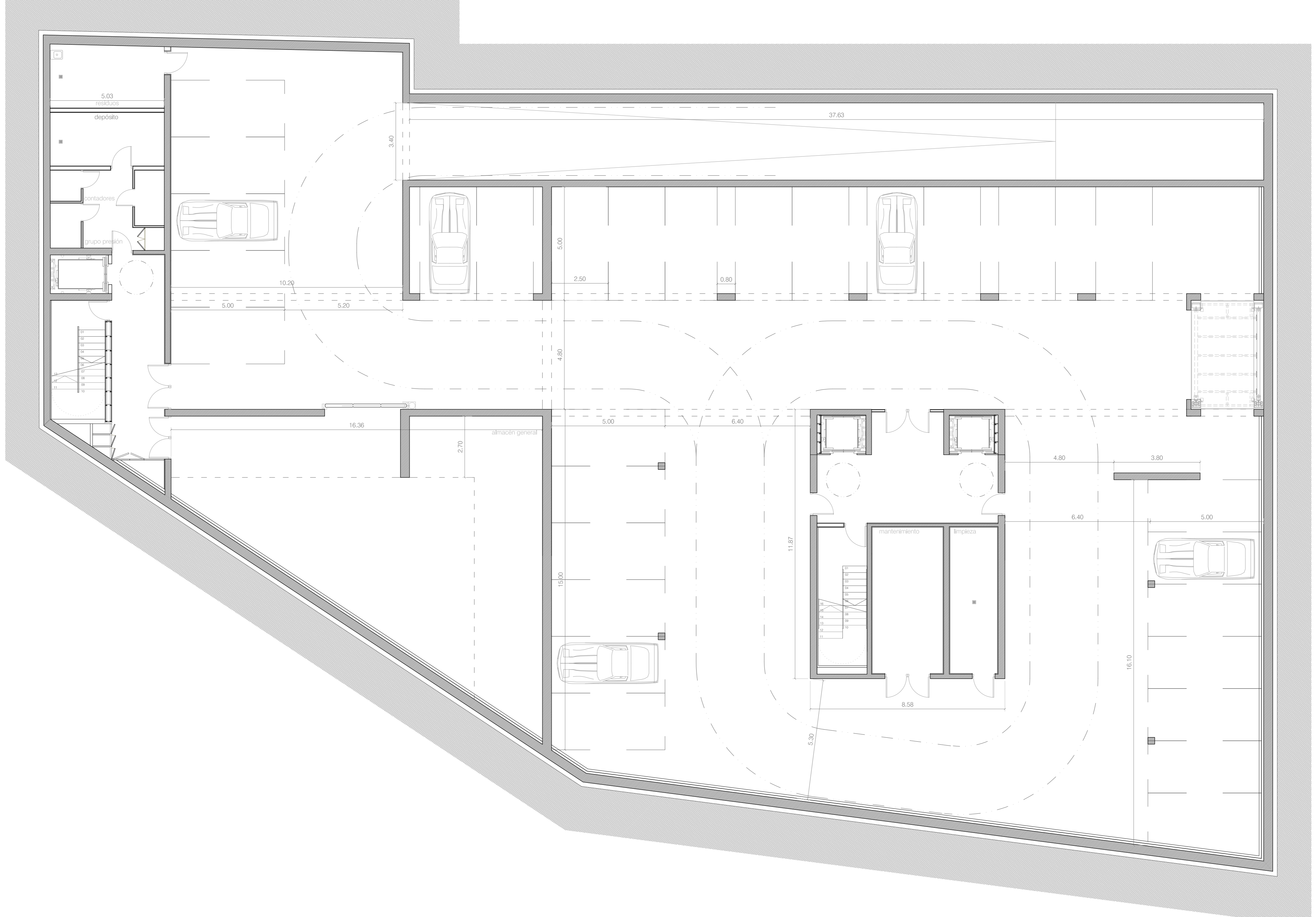
PLANTA SOTANO 2
