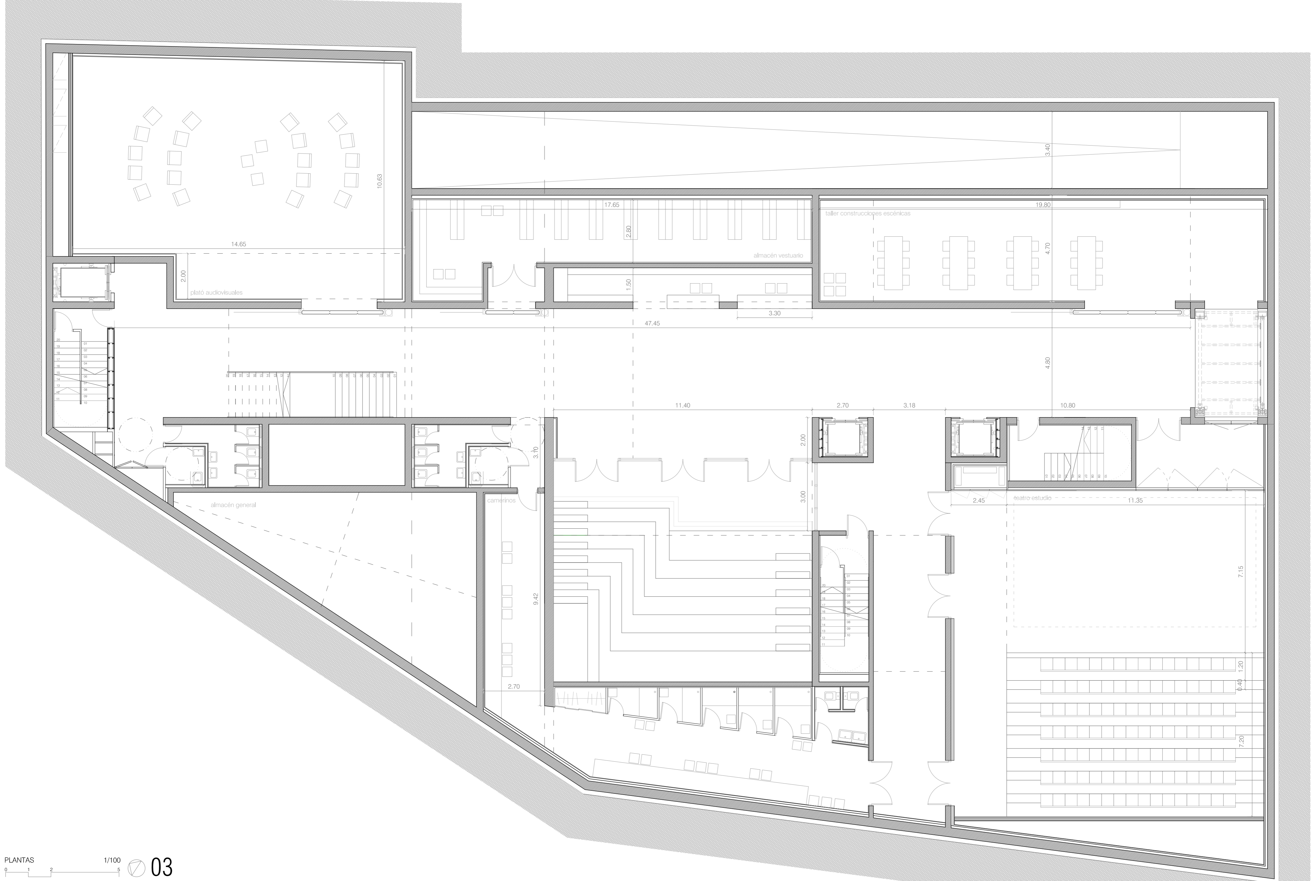
PLANTA SOTANO 1
