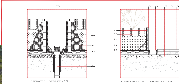
DRENATGE HORTS E: 1/20
