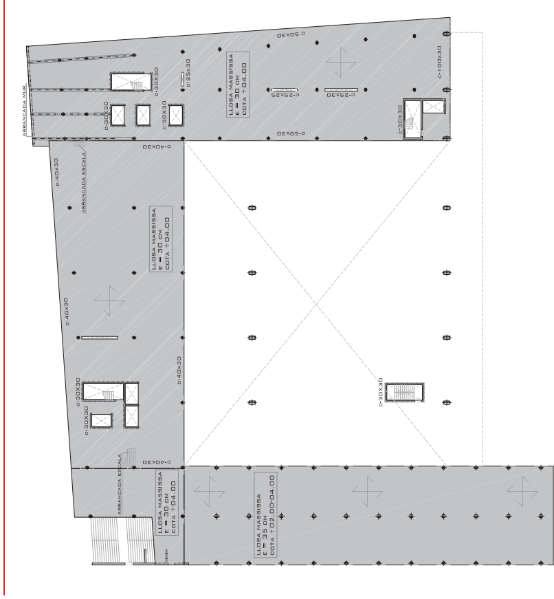
PLANTA SOSTRE PB COTA +04,00
