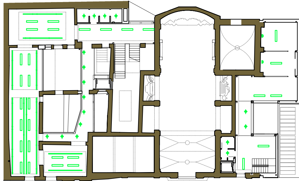
Planta primera
