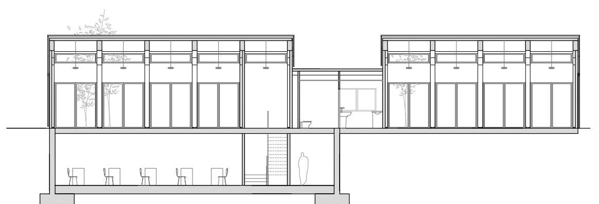
SECCIÓ C-C' MÒDUL TALLER I AULES e 1/100
