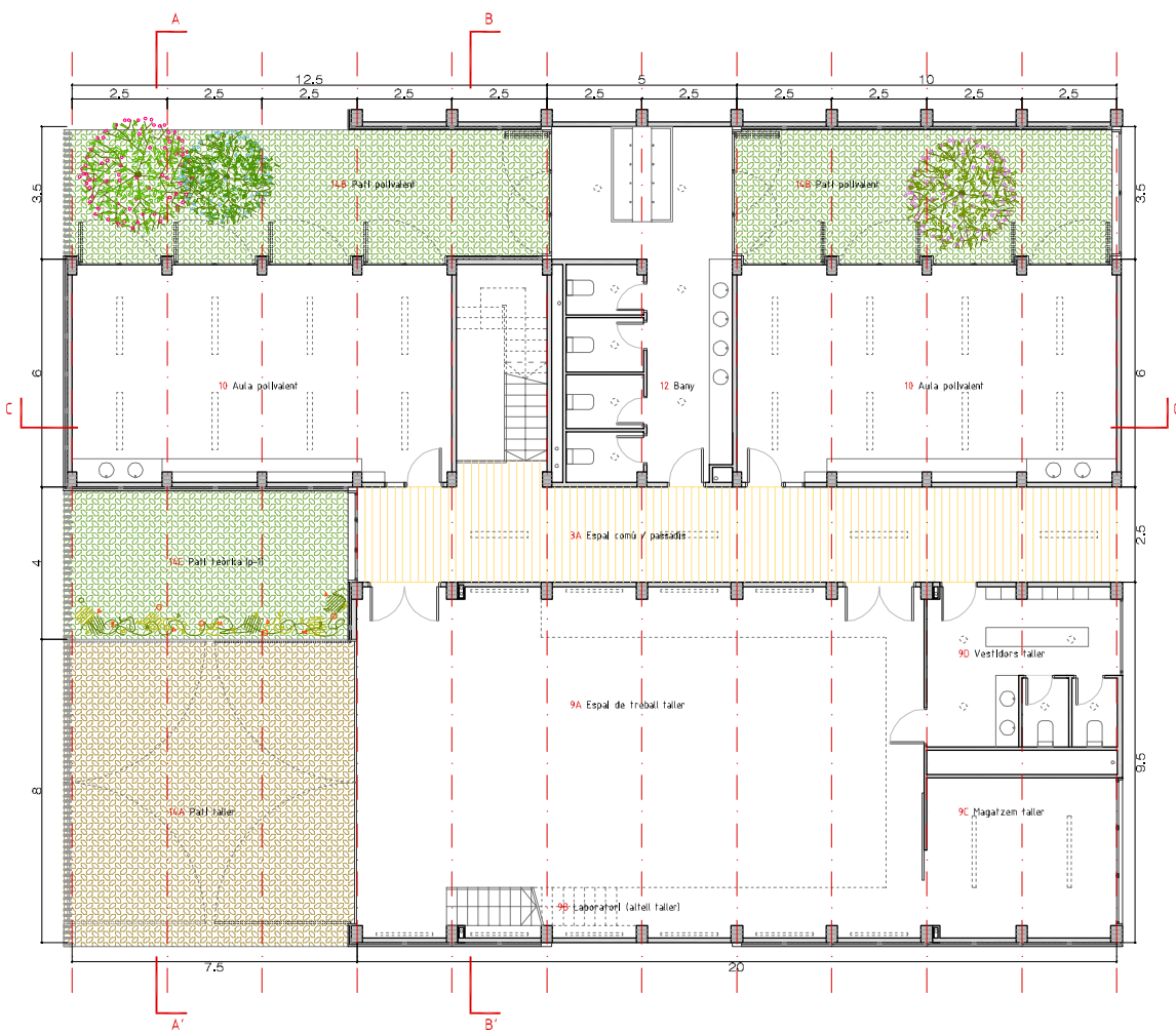
PLANTA BAIXA MÒDUL TALLER I AULES e 1/100
