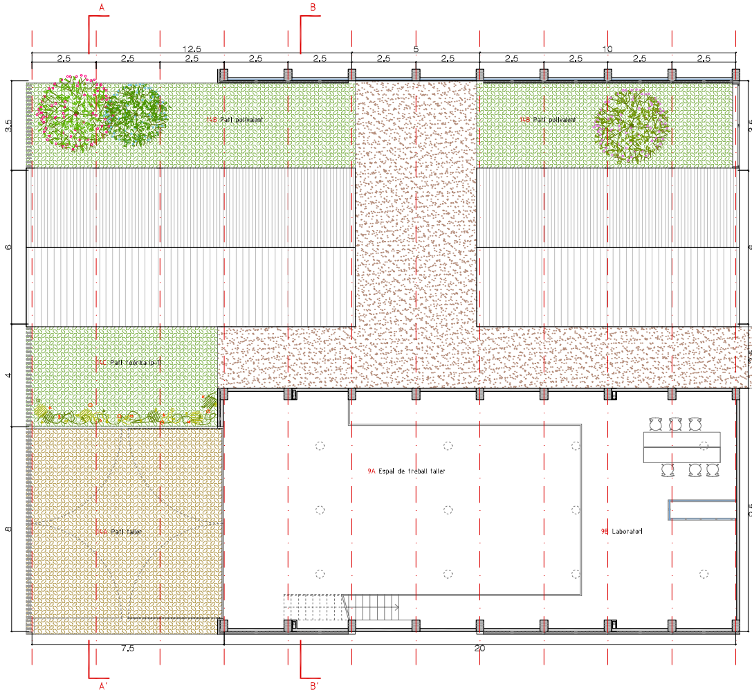
PLANTA ALTELL MÒDUL TALLER I AULES e 1/100
