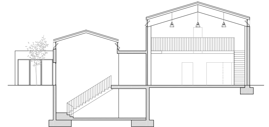
SECCIÓ B-B' MÒDUL TALLER I AULES e 1/100
