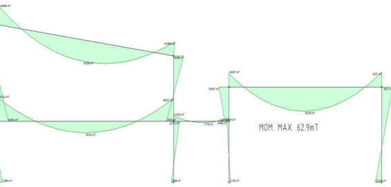
RESULTADOS MOMENTOS ELU
