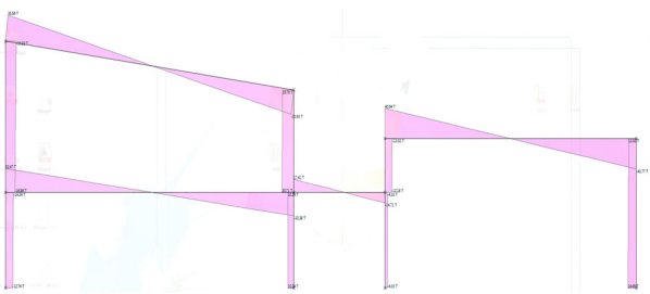
RESULTADOS CORTANTES ELU
