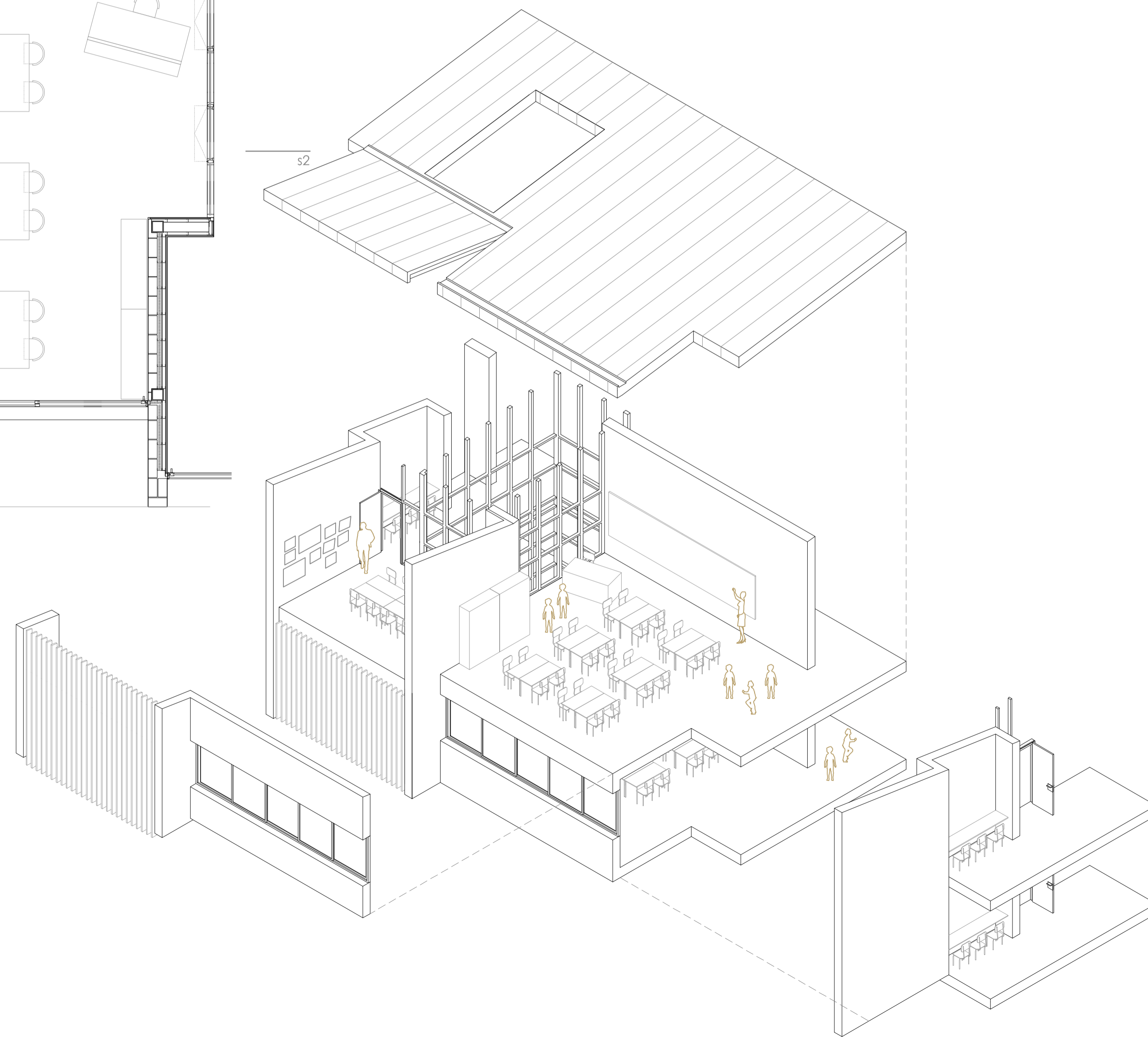
AXONOMETRIA EXPLOTADA
