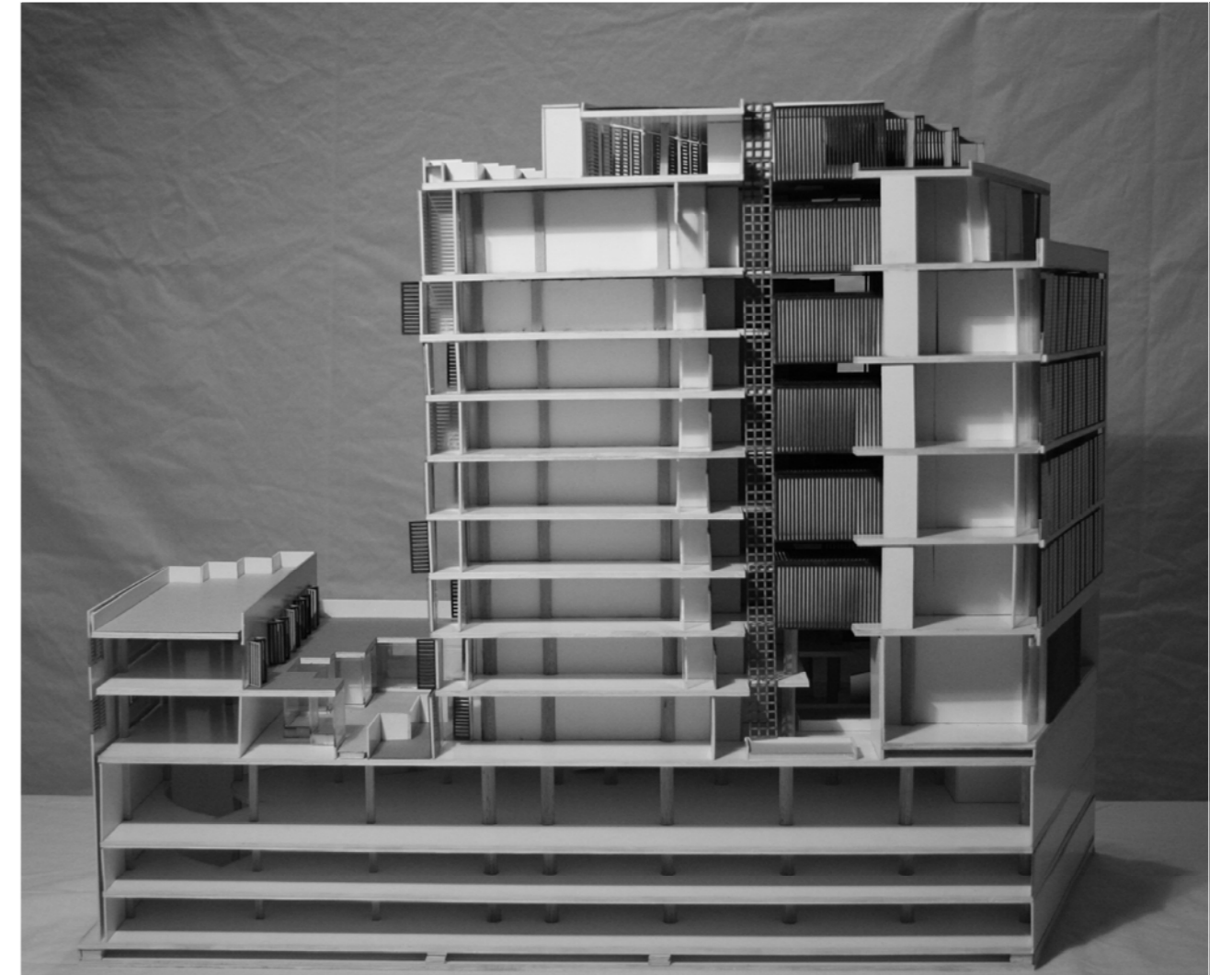
■ SECCIÓ GENERAL PEL PATI INTERIOR
