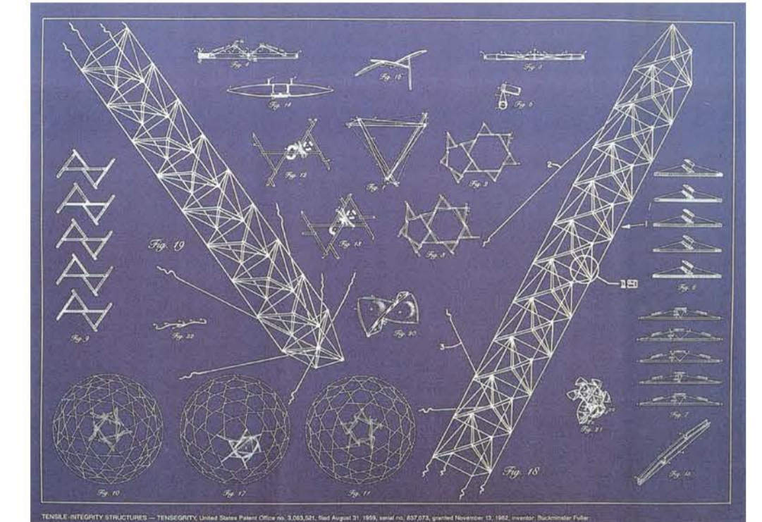
Patent de sistema resistent TANSEGRITY R. Buckminster Fuller. 1959
