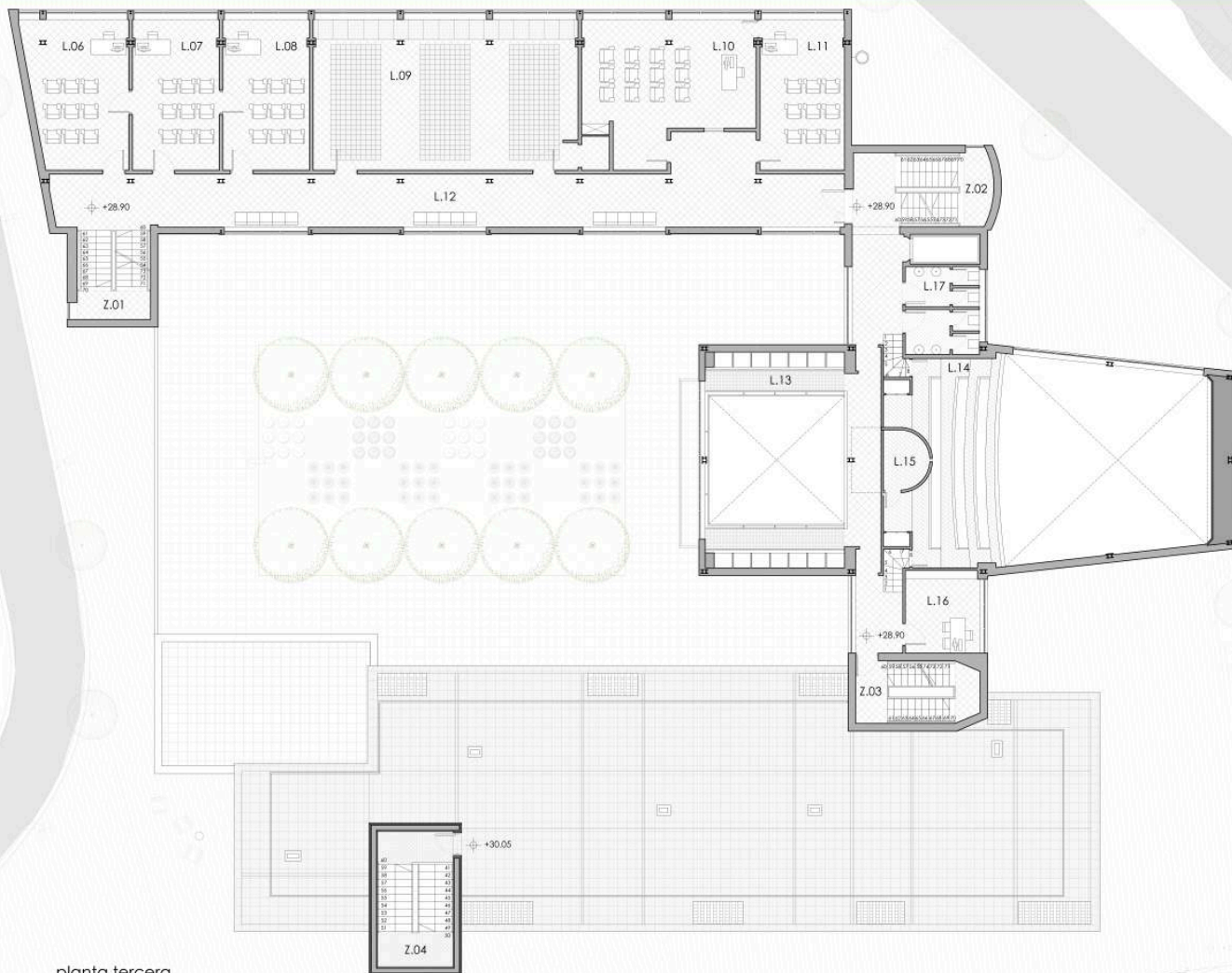
planta tercera
