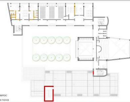
enderroc i obra nova: planta tercera
