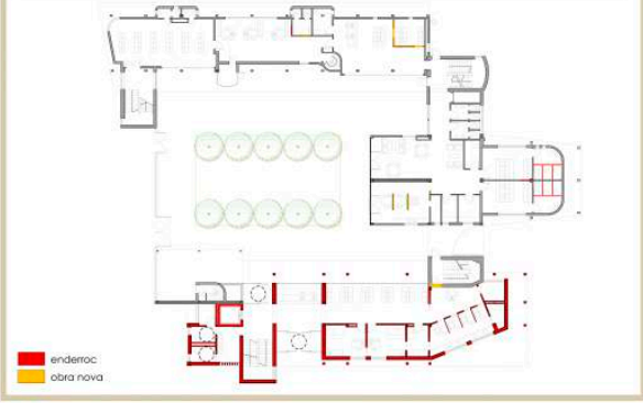
enderroc i obra nova: planta baixa
