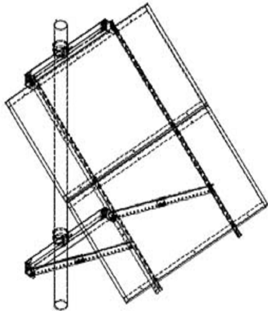
Suport per a 2 panells solars.
